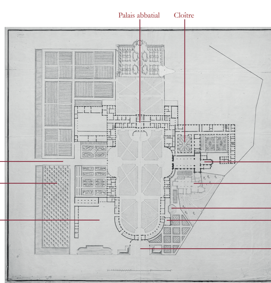
Plan du projet de Dewez, 1760
