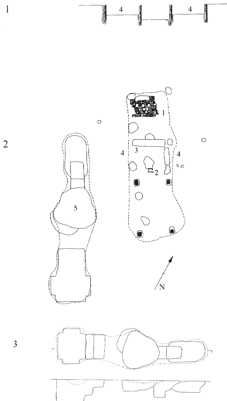
Fig. 4. Plan du mithraeum : 1. Coupe ; 2. Plan : 1) Sol, 2) Conteneur, 3) Fosses, 4) Bancs et fosses, 5) Structure rectangulaire et fosses ; 3. Fosses : coupe.
