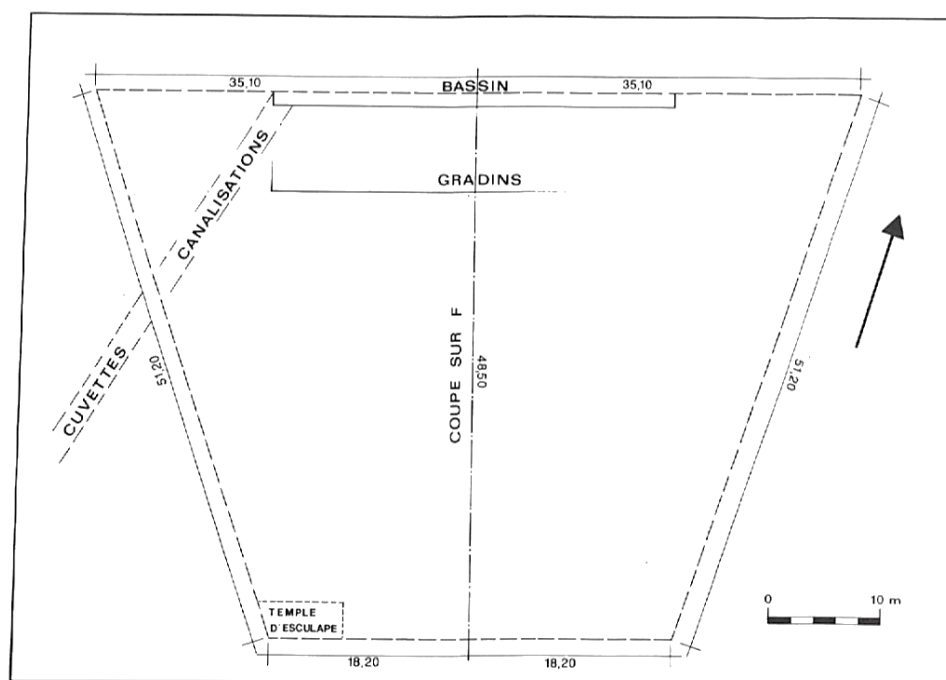
Fig. 6. Plan trapézoïdal de l'asclépiéion.
