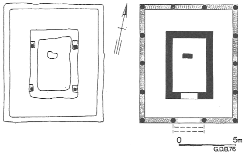
Fig. 5. Les quatre trous de poteaux du bâtiment en bois à cella et reconstitution du Temple B.
