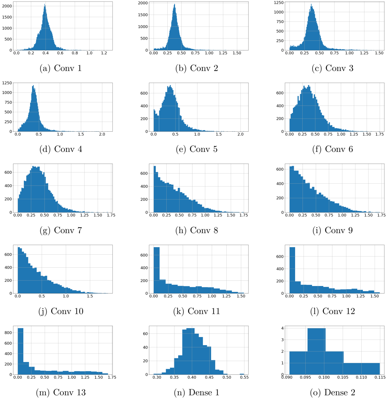
FIGURE A.8 – Réseau Layca 0. L'axe horizontal représente la valeur de l'activation, et l'axe vertical son occurrence dans la couche.
