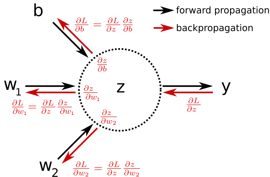
FIGURE 4.5 – Back-propagation dans le neurone : On voit ici que le gradient sur la sortie y est propagée sur le biais b , ainsi que sur chacun des poids w_i .
