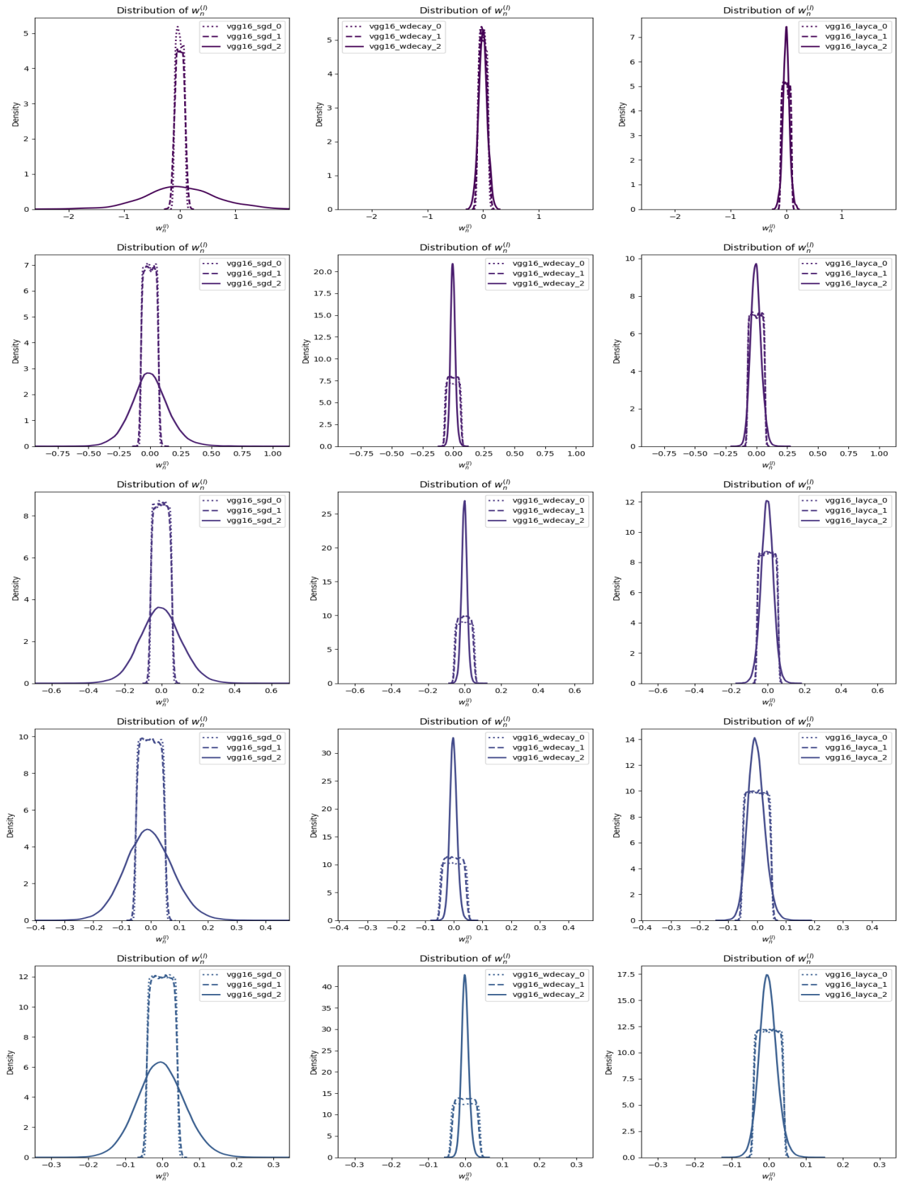
FIGURE 7.8 – Distribution de w_n^{(l)} pour l'ensemble des modèles sur l'ensemble des couches. Les distributions des modèles sgd , weight decay et layca sont respectivement représentées sur la colonne de gauche, du milieu et de droite. La première ligne correspond à la première couche, la deuxième ligne à la deuxième couche, etc.
