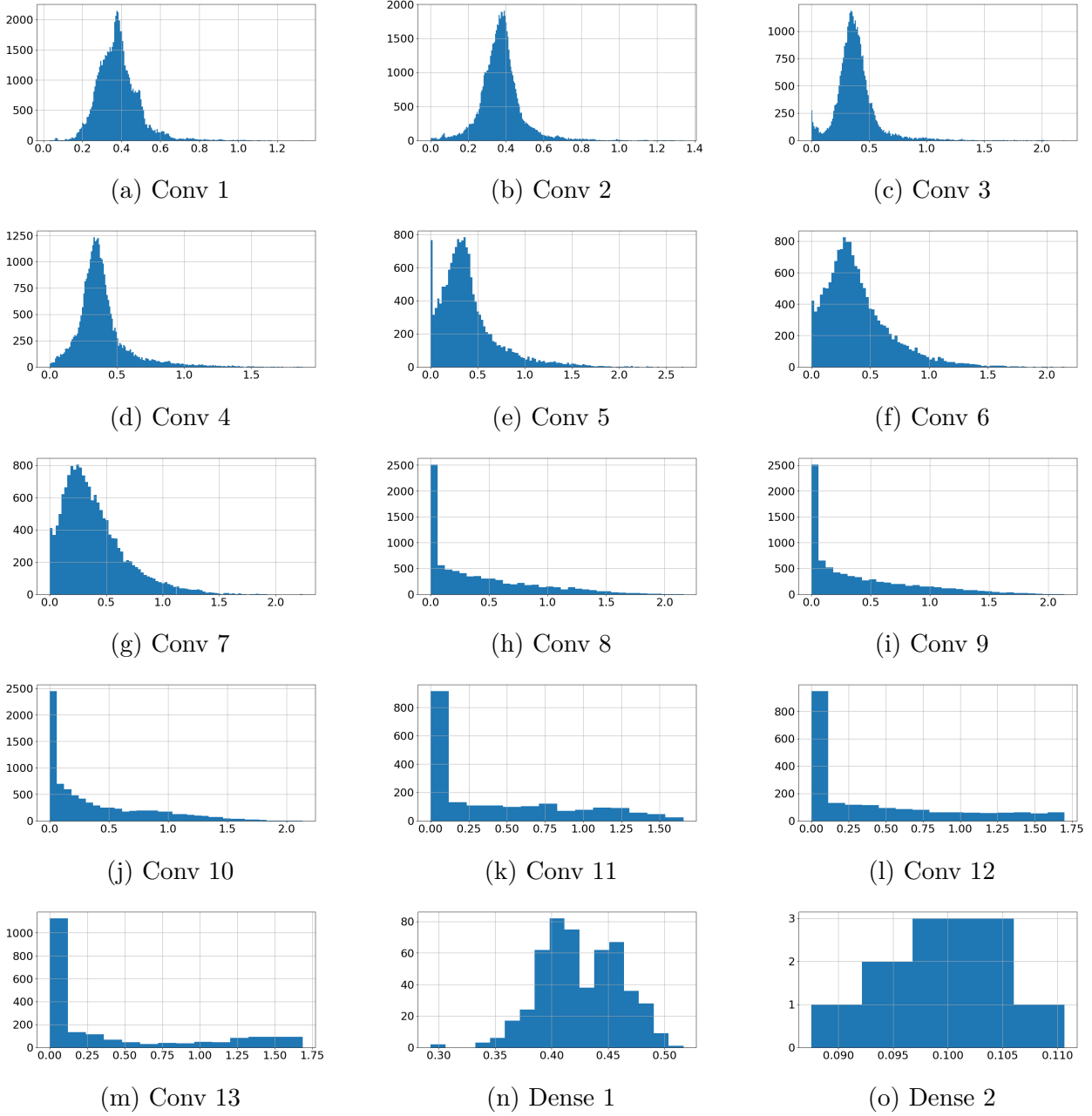
FIGURE A.4 – Réseau SGD 2. L'axe horizontale représente la valeur de l'activation, et l'axe verticale son occurrence dans la couche.
