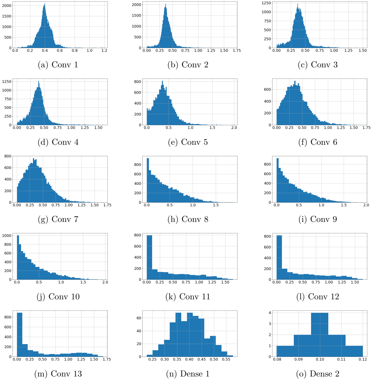
FIGURE A.2 – Réseau SGD 0. L'axe horizontal représente la valeur de l'activation, et l'axe verticale son occurrence dans la couche.
