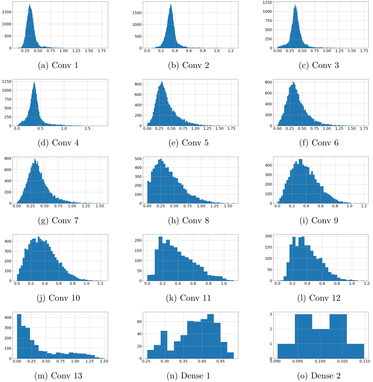
FIGURE A.10 – Réseau Layca 2. L'axe horizontal représente la valeur de l'activation, et l'axe verticale son occurrence dans la couche.
