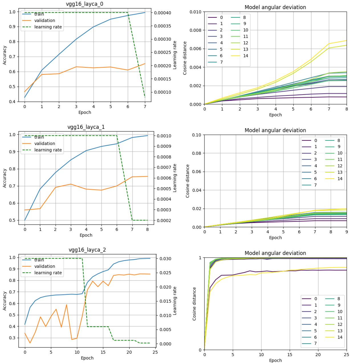
FIGURE 6.6 – Évolution des caractéristiques des modèles entraînés par layca au fil des epochs . Les images de gauche montrent l'évolution de la training (bleu) et validation accuracy (orange) ainsi que du learning rate (vert) du moins bon au meilleur modèle. Les images de droite montrent l'évolution de la cosinus distance des couches au fil des epochs . Les numéros des couches correspondent aux numéros de la FIGURE 6.2 moins un.
