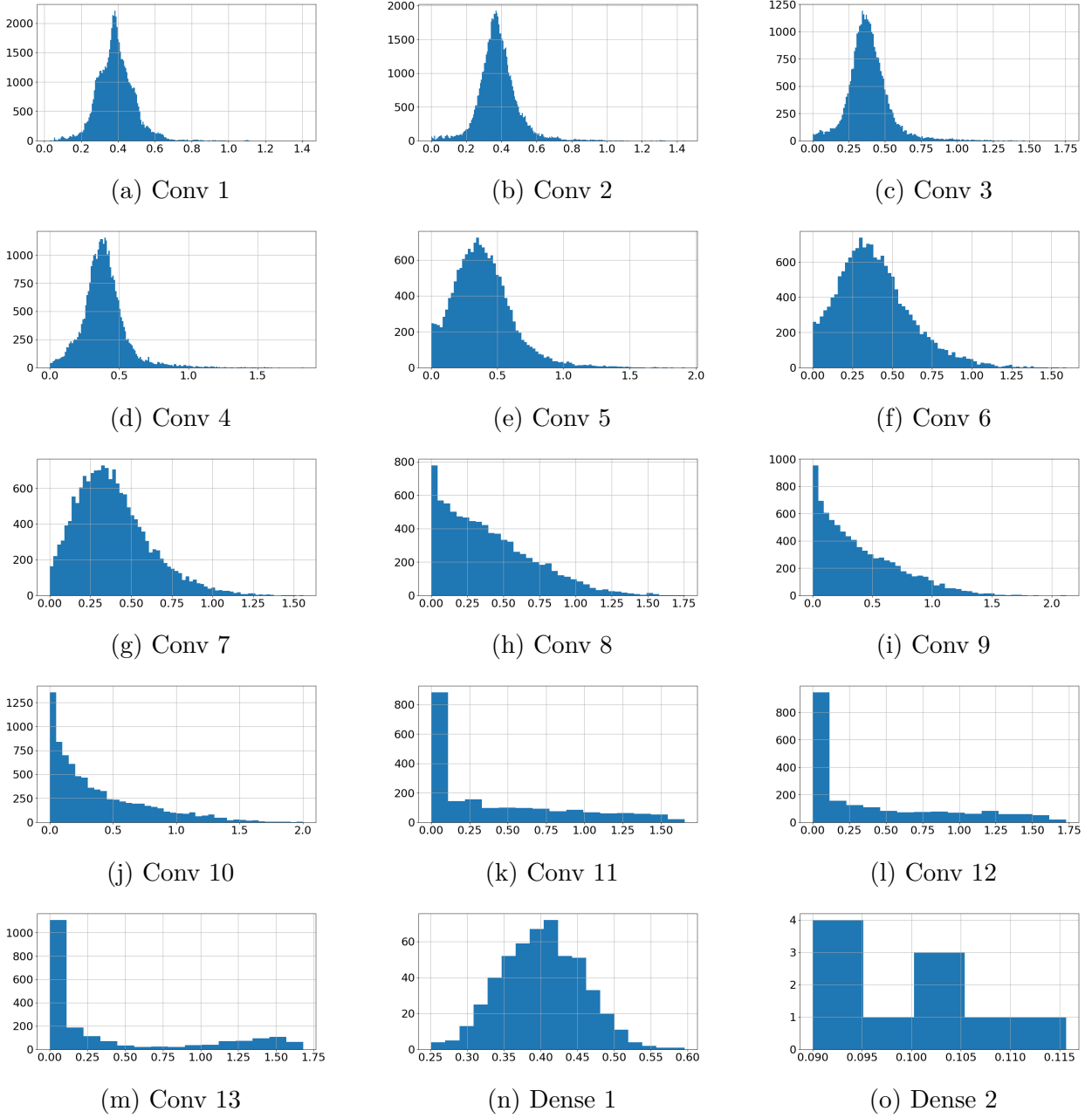
FIGURE A.3 – Réseau SGD 1. L'axe horizontal représente la valeur de l'activation, et l'axe verticale son occurrence dans la couche.
