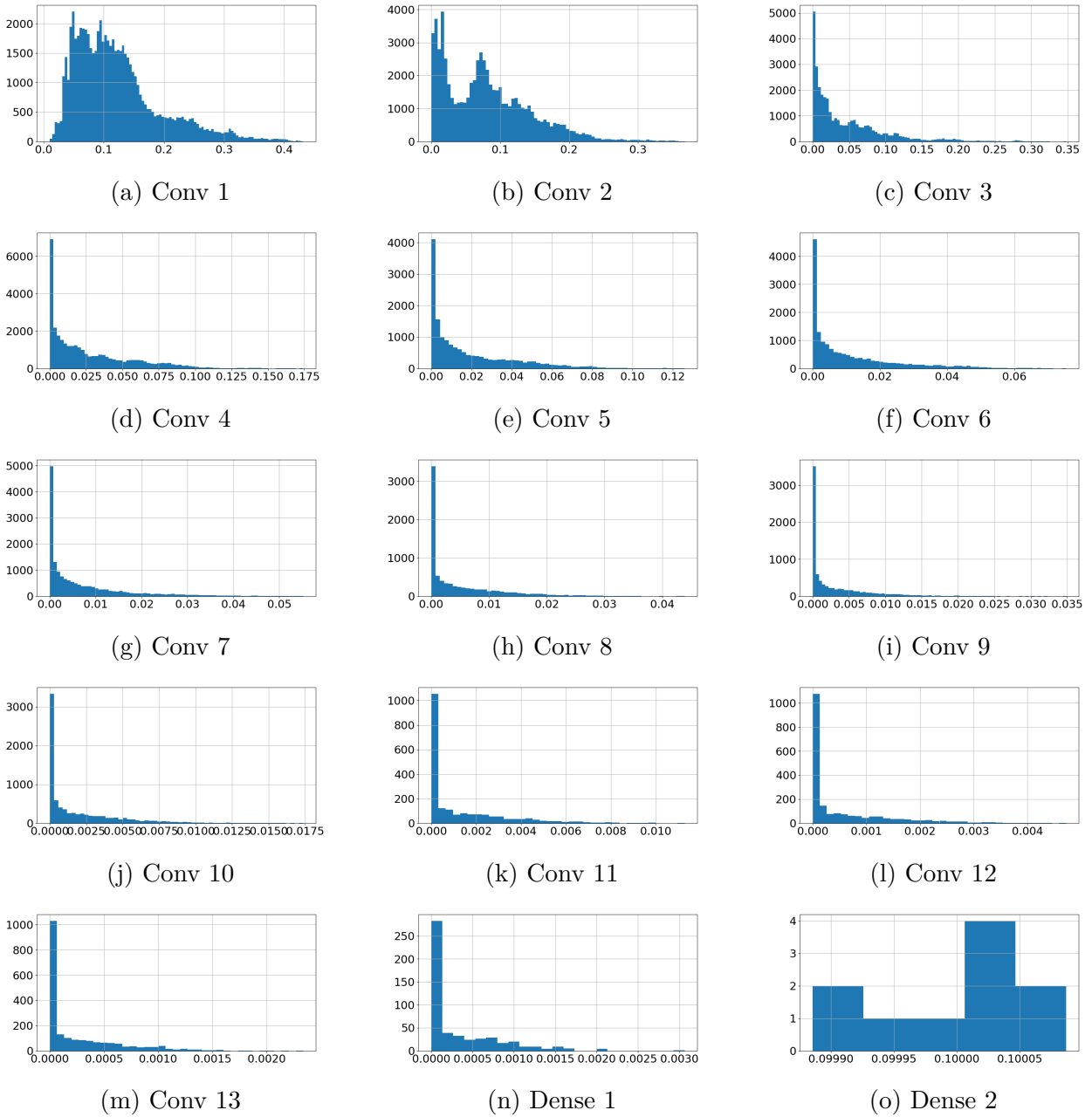
FIGURE A.1 – Réseau Initial. L'axe horizontale représente la valeur de l'activation, et l'axe verticale son occurrence dans la couche.
