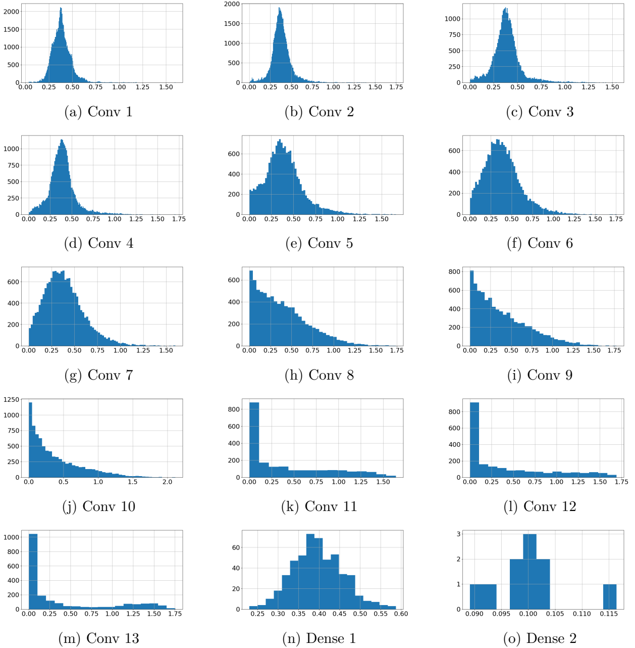
FIGURE A.6 – Réseau WD 1. L'axe horizontal représente la valeur de l'activation, et l'axe verticale son occurrence dans la couche.
