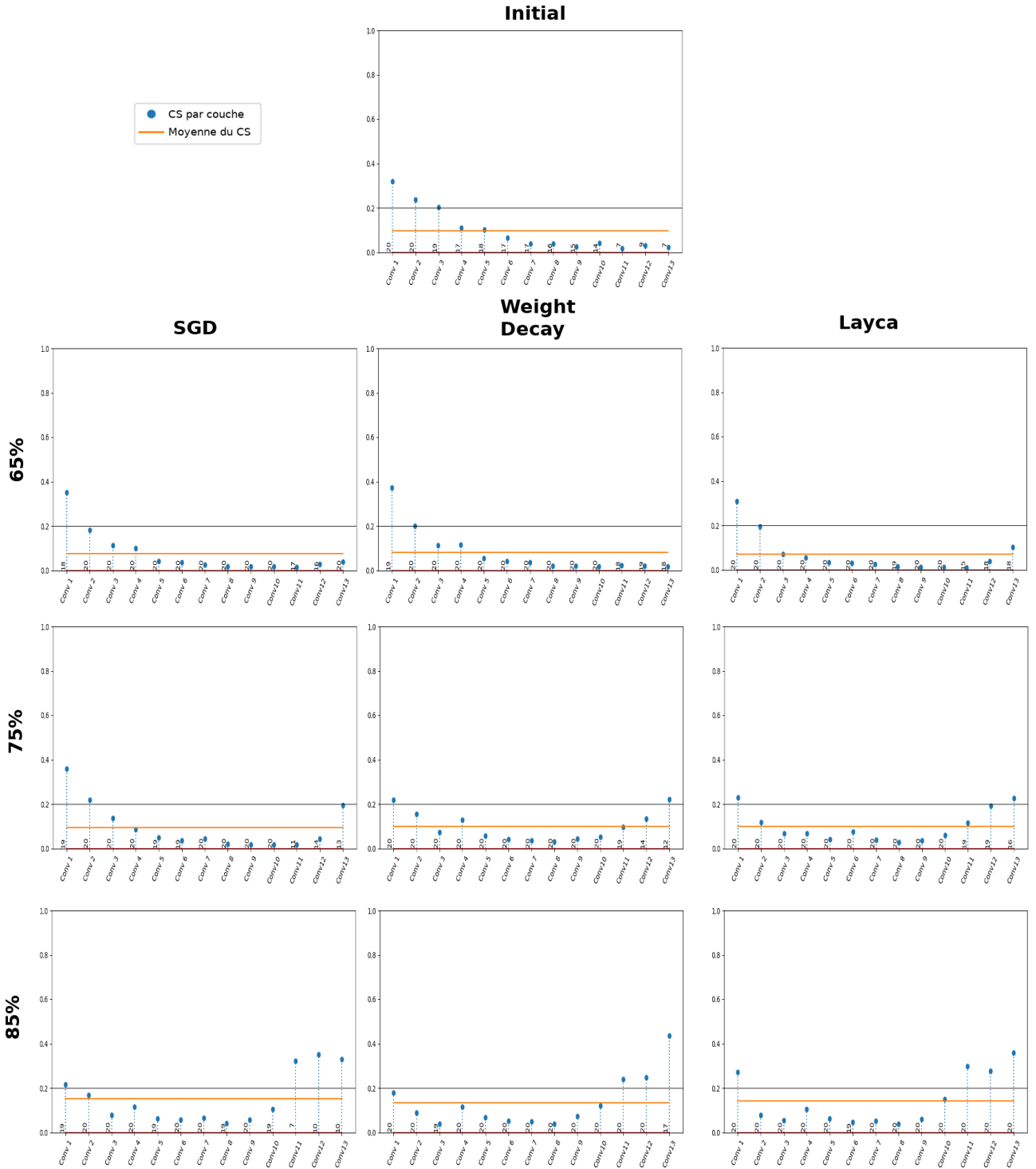
FIGURE 8.9 – Coefficient de silhouette par couche pour Ratio1=0.1, Ratio2=0.2, Dist=Cosine, 1000 images d'activation et 20 neurones
