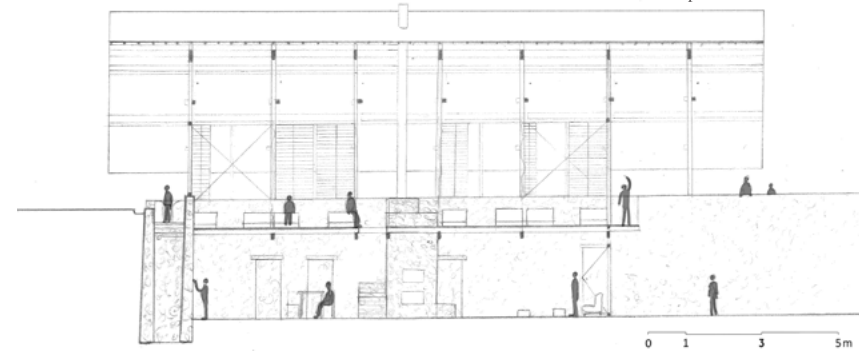
Coupe longitudinale : le rez-de-chaussée est exprimé dans la masse des murs, l'étage profite d'une structure plus légère.
