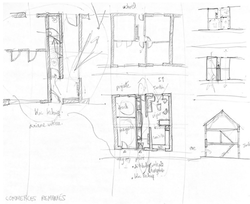
Esquisses de dissociation de commerce-logement : exemple de la maison de Mémé Nicole.
