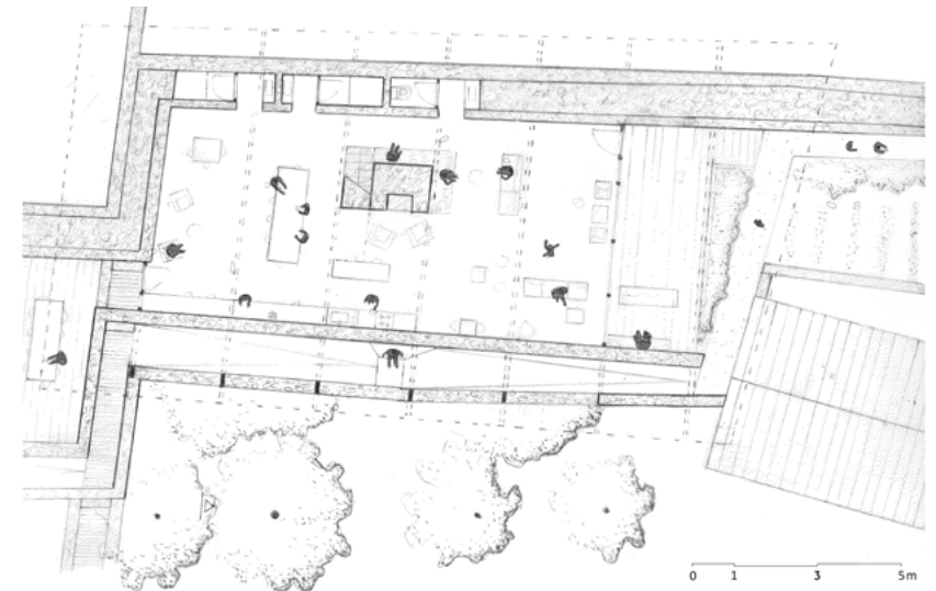
Plan du rez-de-chaussée : l'espace intérieur est entouré de la circulation publique. Un poêle de masse occupe le centre de l'espace.
