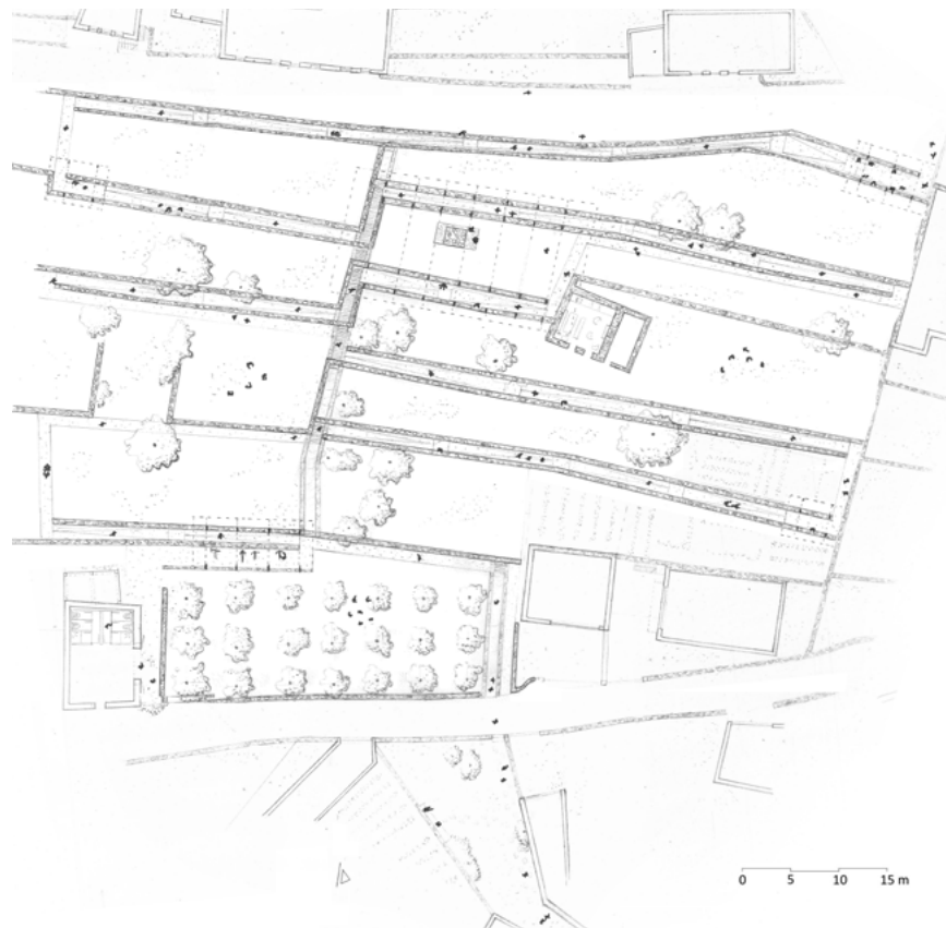
Plan de l'état projeté : le parcours s'effectue dans une double épaisseur de murs.
