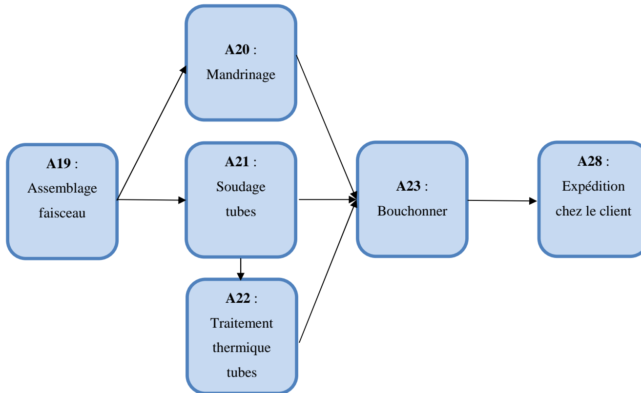
Figure 27: Processus de fourniture de faisceau de rechange (deuxième partie)
