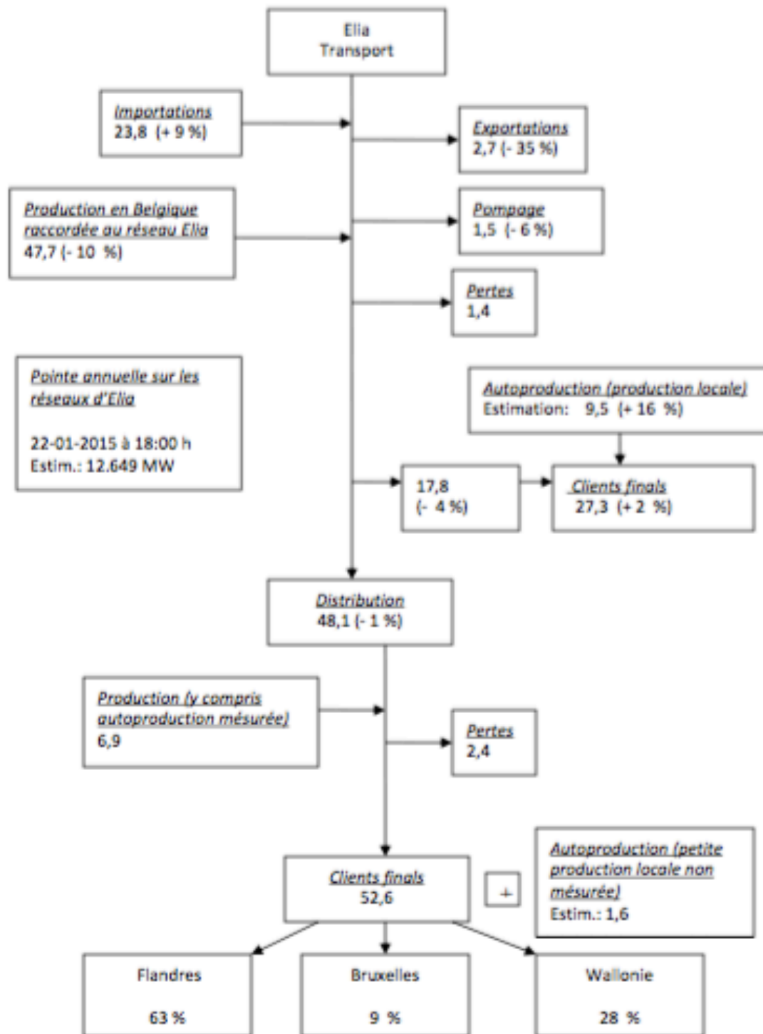
FLUX D'ELECTRICITE EN BELGIQUE EN 2015 (en TWh) (± ... %) = variations par rapport à 2014
