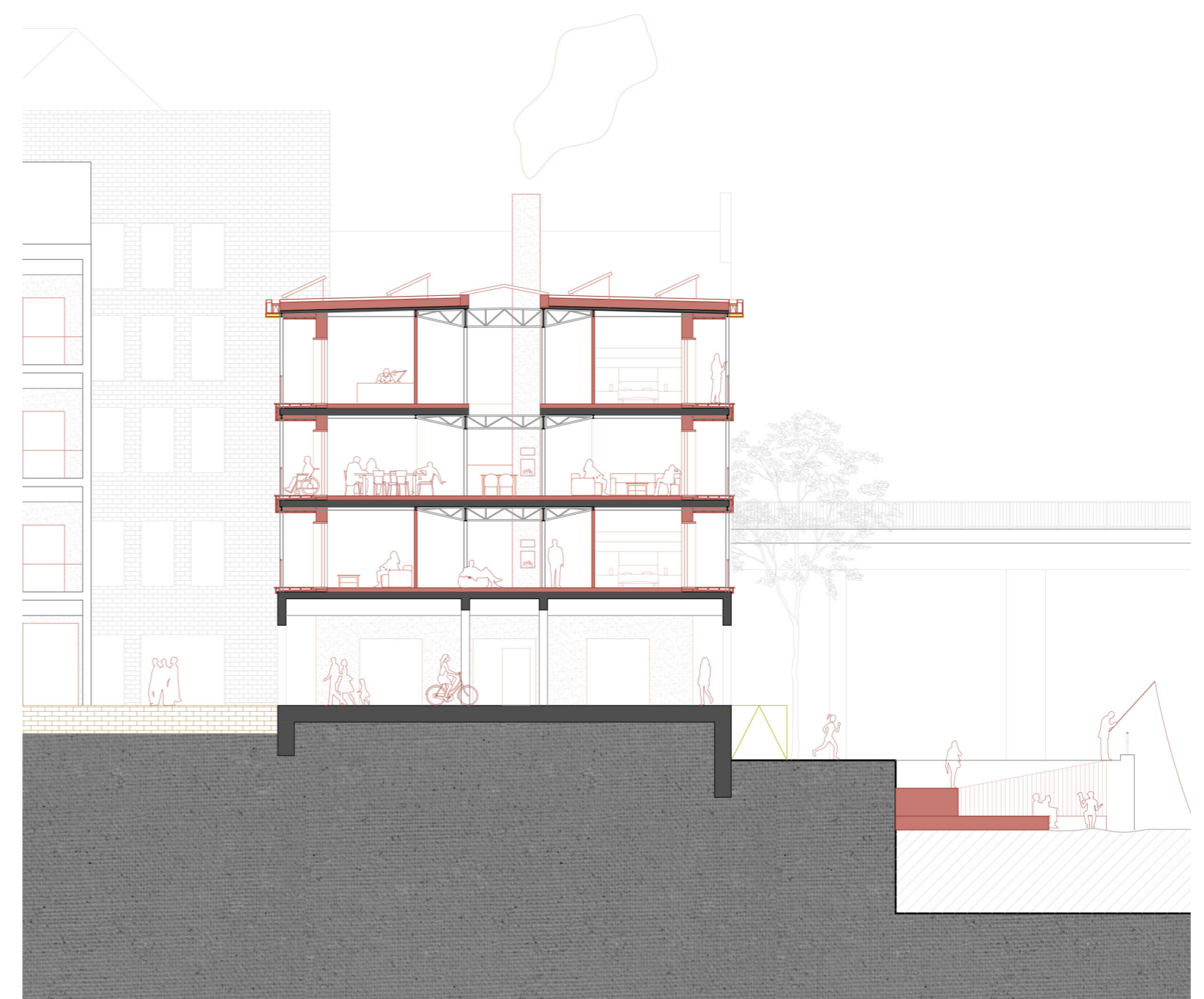
Coupe Bâtiment 1
