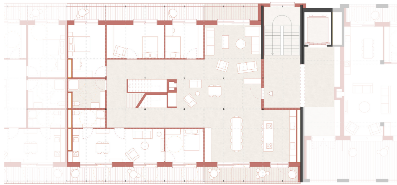
R+2 Bâtiment 1
