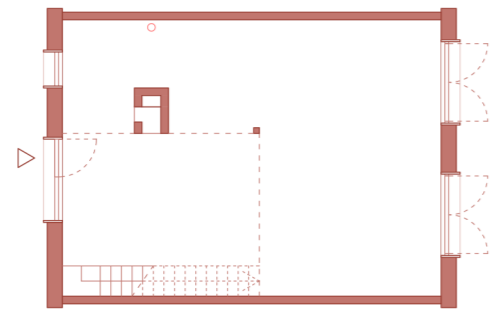
RDC Aménagement sans cloisonnement
