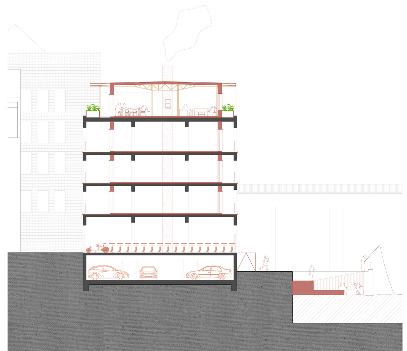
Coupe Bâtiment 4
