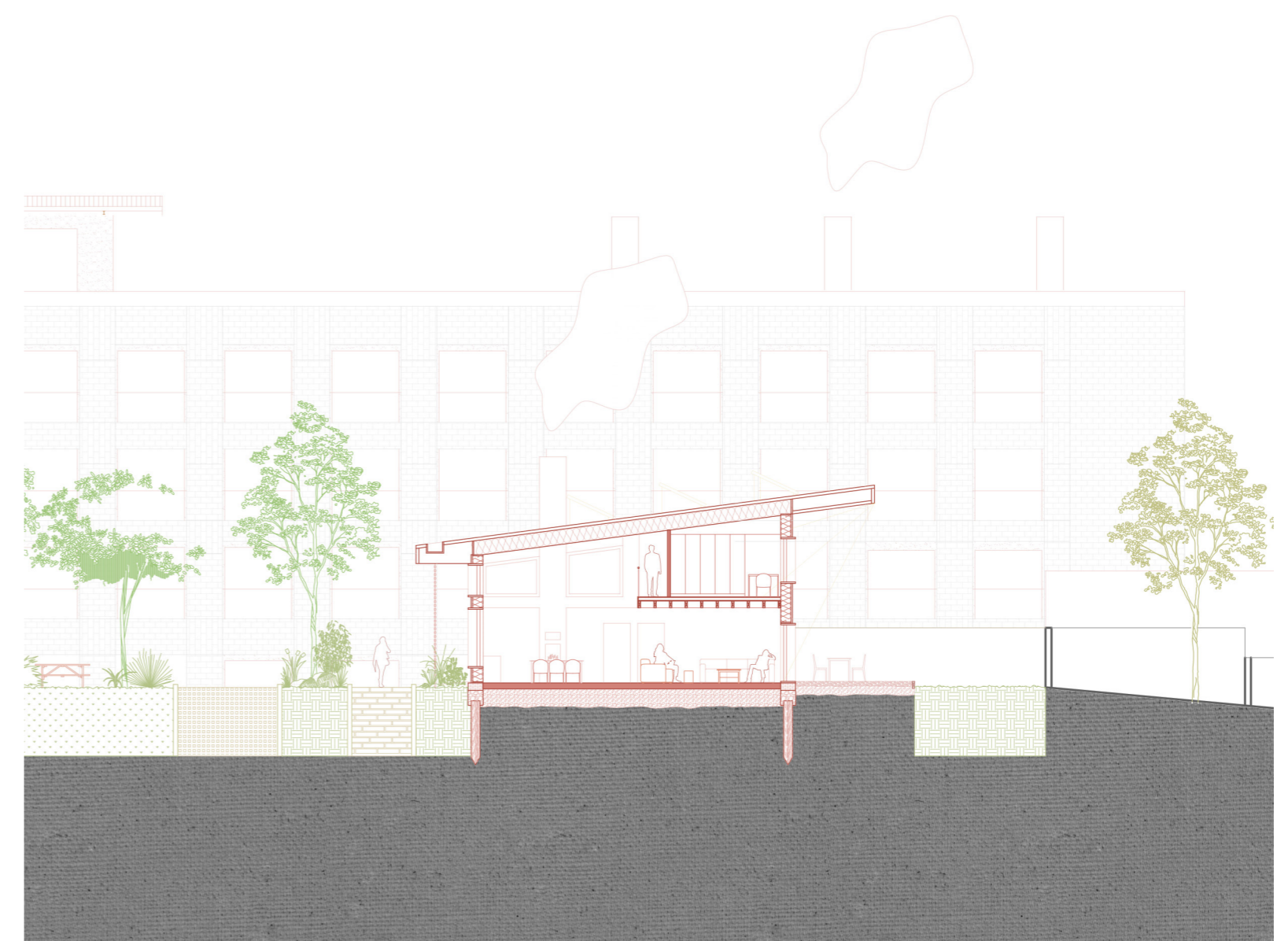
Coupe Maison mitoyenne
