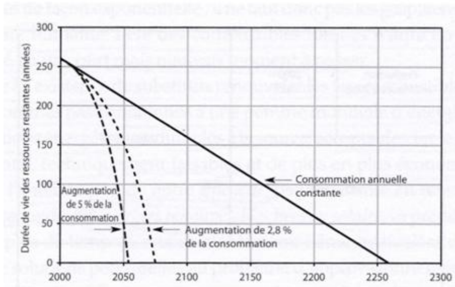
Figure I.7 : Durée de vie des ressources restantes de gaz naturel
