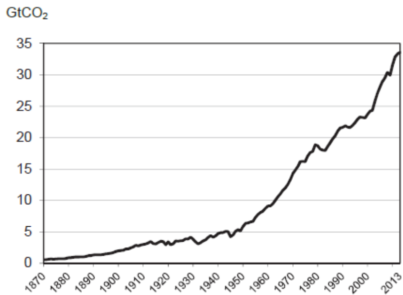
Figure I.9 : Evolution des émissions de CO 2 provenant de la combustion des énergies fossiles, 1870-2013
