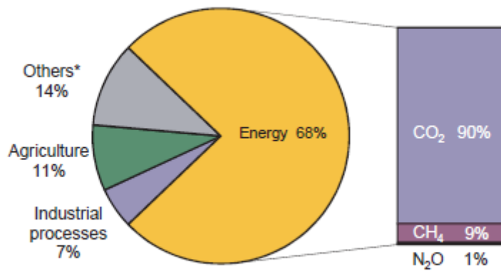
Figure I.8 : Répartition des émissions anthropiques de GES
