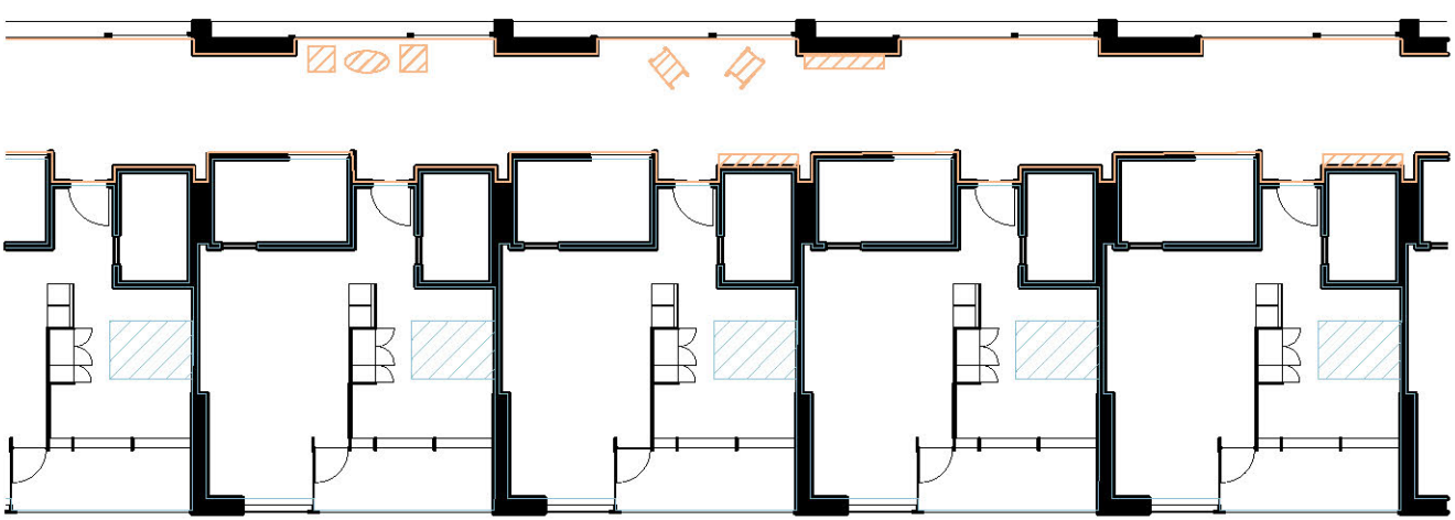
Peter Zumthor, Résidence pour seniors, Suisse, 1993
