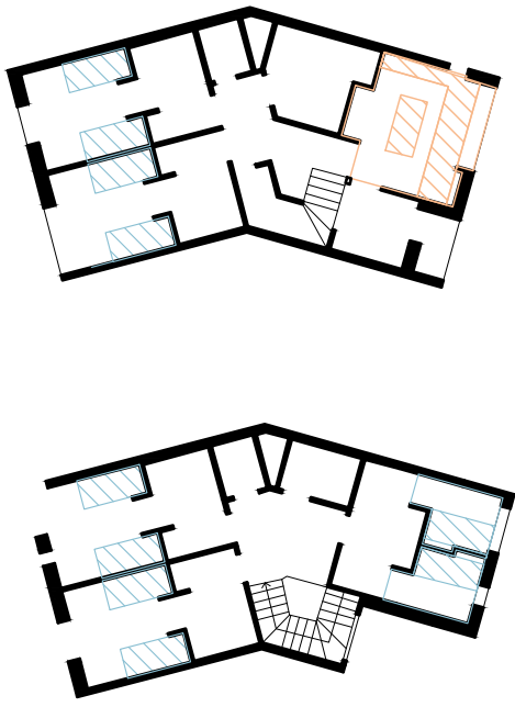
ASAS Arkitektur, Folkhøgskole Student Housing, Norvège, 2014
