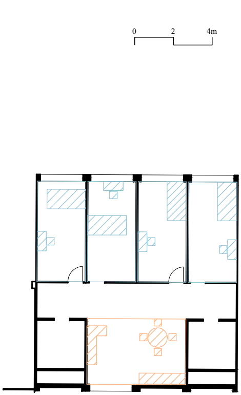
Willy Van der Meeren, Logements pour étudiants de la VUB, Belgique, 1956
