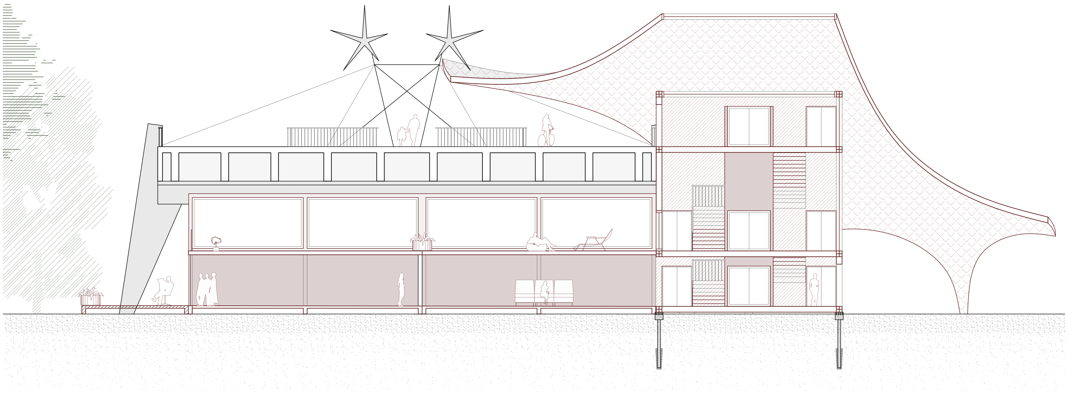
COUPE B-B'
