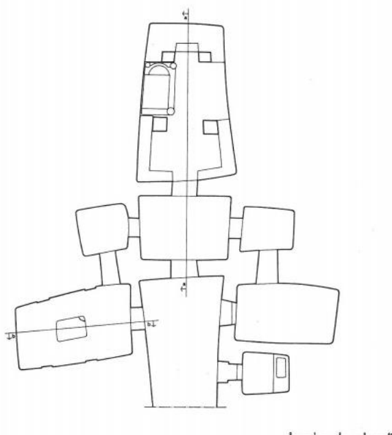
FIG. 96. San Giuliano, necropoli di Chiusa Cima. Tumulo Cima. Plan de la tombe principale. Troisième quart du VII e s. av. J. -C (STEINGRÄBER 2009b, p. 263).
