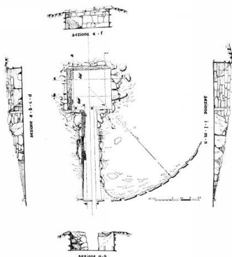
FIG. 57. Vetulonia, necropoli di Val Berretta. Tumulo I. Plan et section. Seconde moitié du VI e voire début du V e s. av. J. -C. (BOGLIONE 2009, p. 28).
