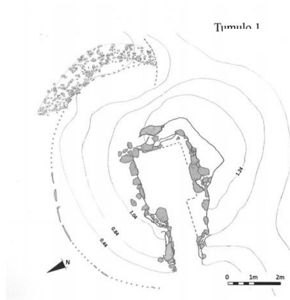
FIG. 62. Vetulonia, necropoli di Santa Teresa. Tumulo I. Plan. Fin VII e – première moitié du VI e s. av. J. -C. (BOGLIONE 2009, p. 52).
