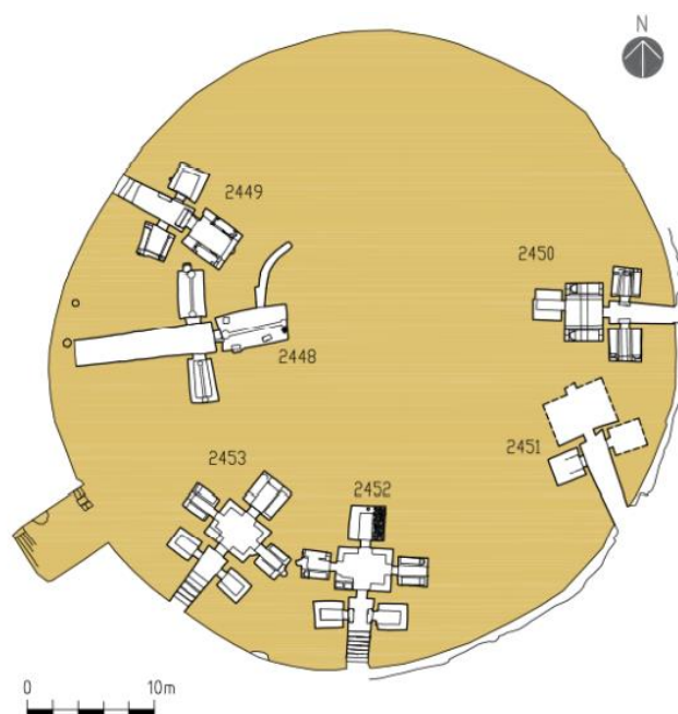
FIG. 111. Caere, Campo della Fiera . Tumulo di Campo della Fiera . Plan. Première moitié du VII e s. – fin VI e s. av. J. -C. (COSENTINO 2018, p. 346).
