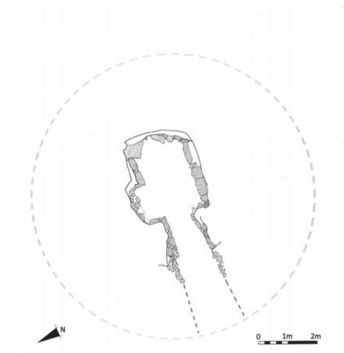
FIG. 64. Vetulonia, necropoli di Santa Teresa. Tumulo IV. Plan. Fin VII e – première moitié du VI e s. av. J. -C. (BOGLIONE 2009, p. 56).
