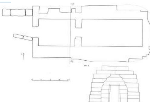
FIG. 91. San Giuliano, necropoli del Caiolo. Cuccumella. Plan et section. VII e s. av. J. -C. (STEINGRÄBER 2009a, p. 53).
