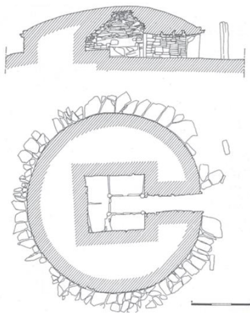
FIG. 47. Populonia, necropoli di Poggio della Porcareccia. Tomba dei Flabelli. Plan et section. VII e – VI e s. av. J. -C. (BIAGI, CAMILI et MILLETTI 2020, p. 295).
