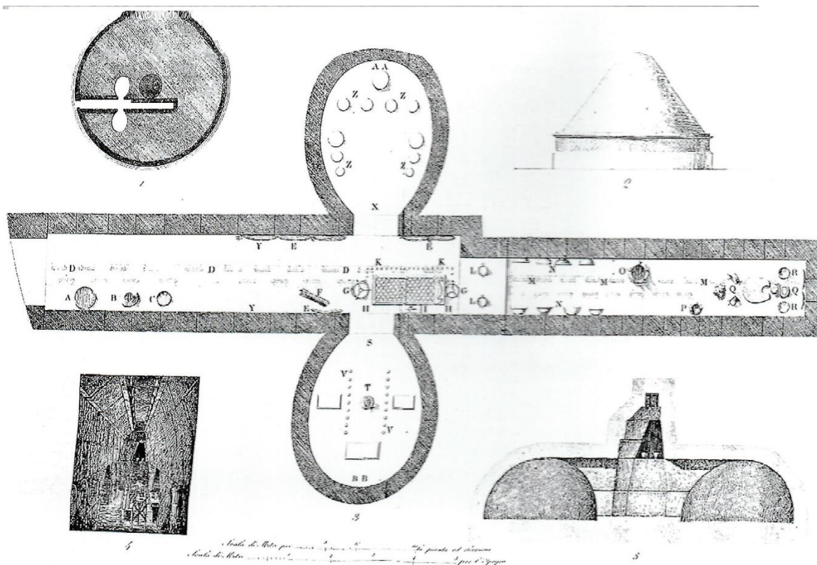
FIG. 113. Caere, necropoli del Sorbo. Tumulo Regolini Galassi. Planimétrie avec la disposition des objets selon Luigi Griffi. VII e s. – VI e s. av. J. -C. (MANDOLESI 2020, p. 20).
