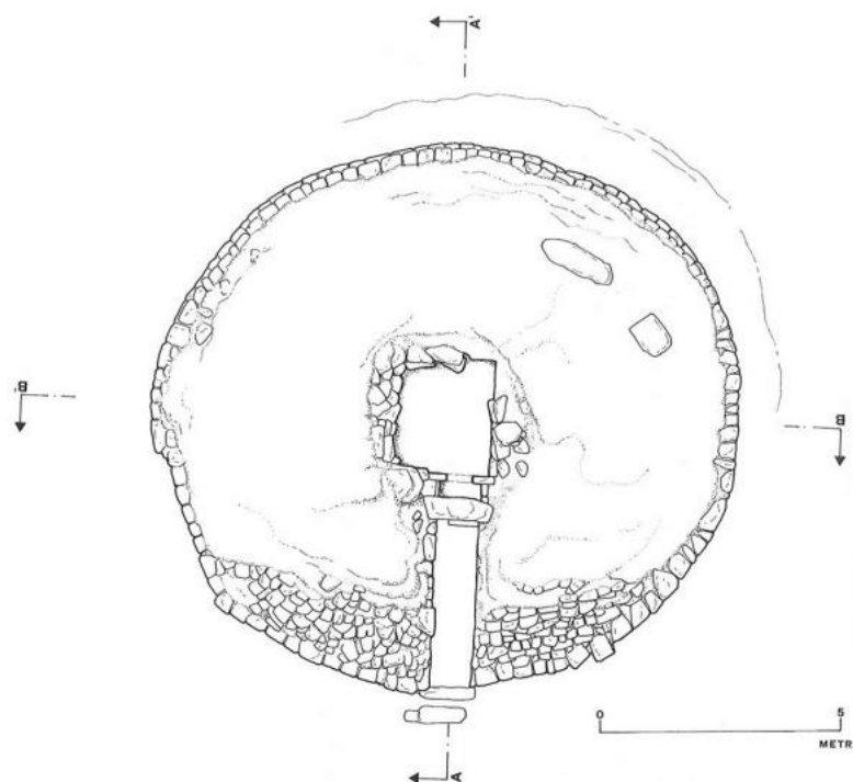
FIG. 60. Vetulonia, necropoli di Val Berretta. Tumulo XIII. Plan. VII e - V e s. av. J. -C. (BOGLIONE 2009, p. 37).
