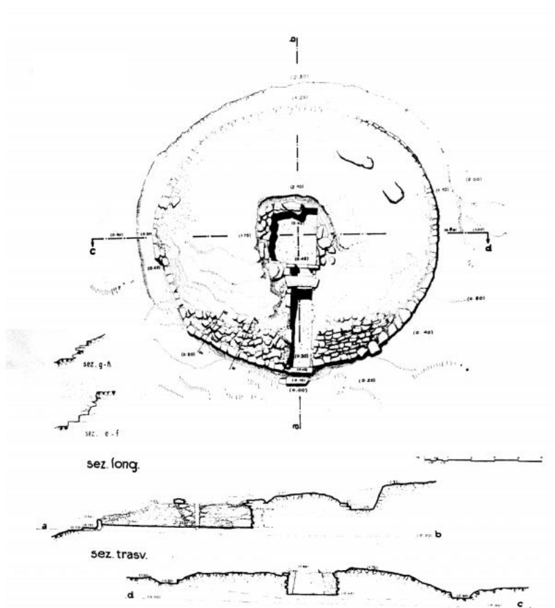
FIG. 61. Vetulonia, necropoli di Val Berretta. Tumulo LVI Plan et section. VI e s av. J. -C. (BOGLIONE 2009, p. 40).
