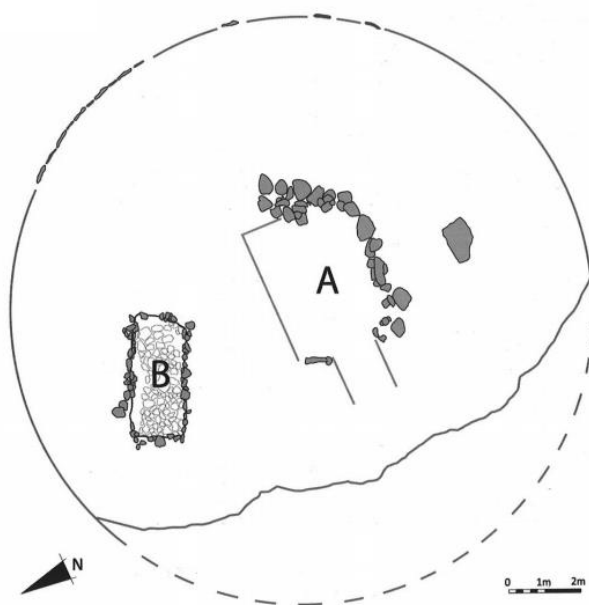
FIG. 65. Vetulonia, necropoli di Santa Teresa. Tumulo V. Plan. Deuxième moitié du VII e s. et fin VII e – première moitié du VI e s. av. J. -C. (BOGLIONE 2009, p. 57).
