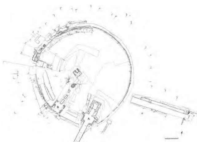
FIG. 76. Vulci, necropoli di Ponte Rotto. Cuccumella. Plan. Dernières décennies du VII e s. av. J. -C. (MORETTI SGUBINI 2015, p. 626).
