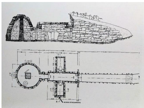
FIG. 27. Quinto Fiorentino. Il Montagnola. Plan et section. Fin VII e s. av. J. -C. (MANDOLESI 2020, p. 71).
