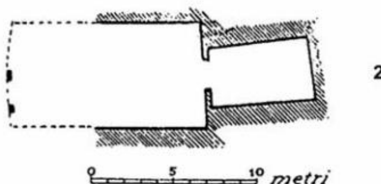
FIG. 86. Tarquinia, necropoli della Doganaccia. Tumulo del Re. Plan. Première moitié du VII e s. av. J. -C. (MANDOLESI 2009a, p. 15).
