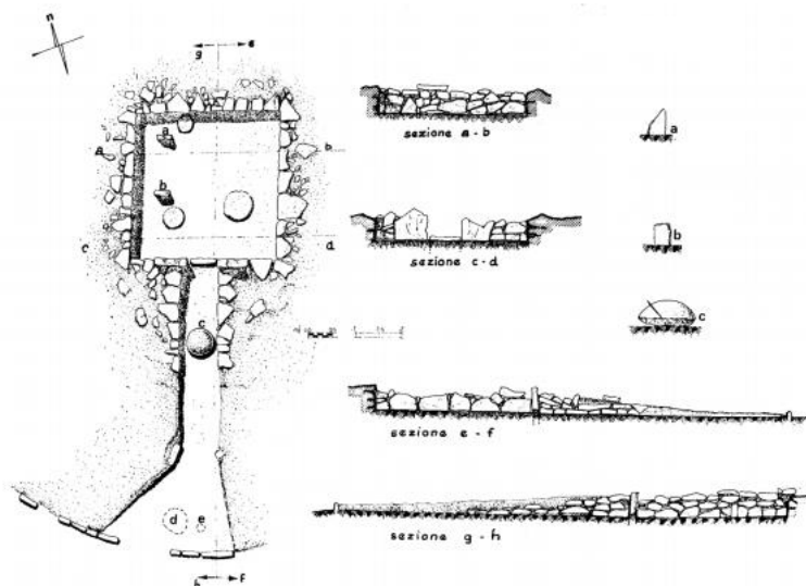
FIG. 58. Vetulonia, necropoli di Val Berretta. Tumulo II. Plan et section. Seconde moitié du VI e voire début du V e s. av. J. -C. (BOGLIONE 2009, p. 30).
