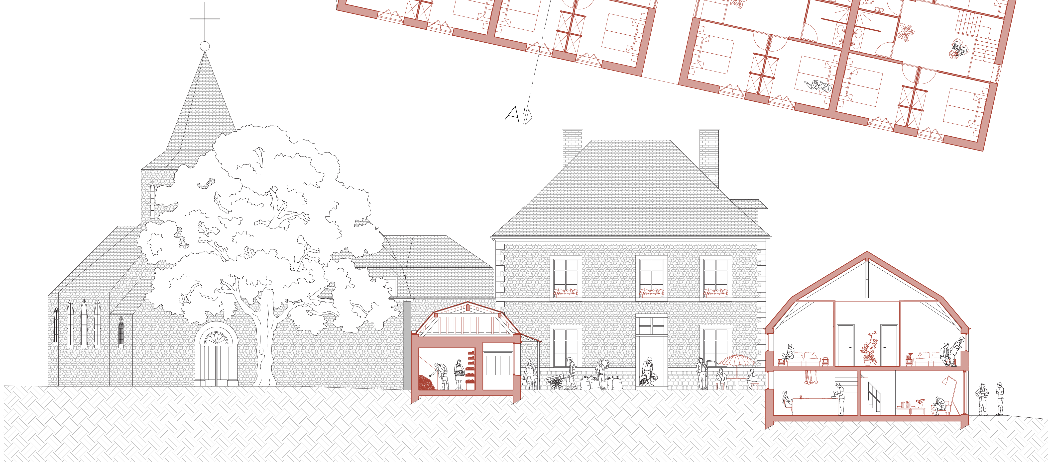
COUPE AA' - ÉCHELLE 1 : 100
