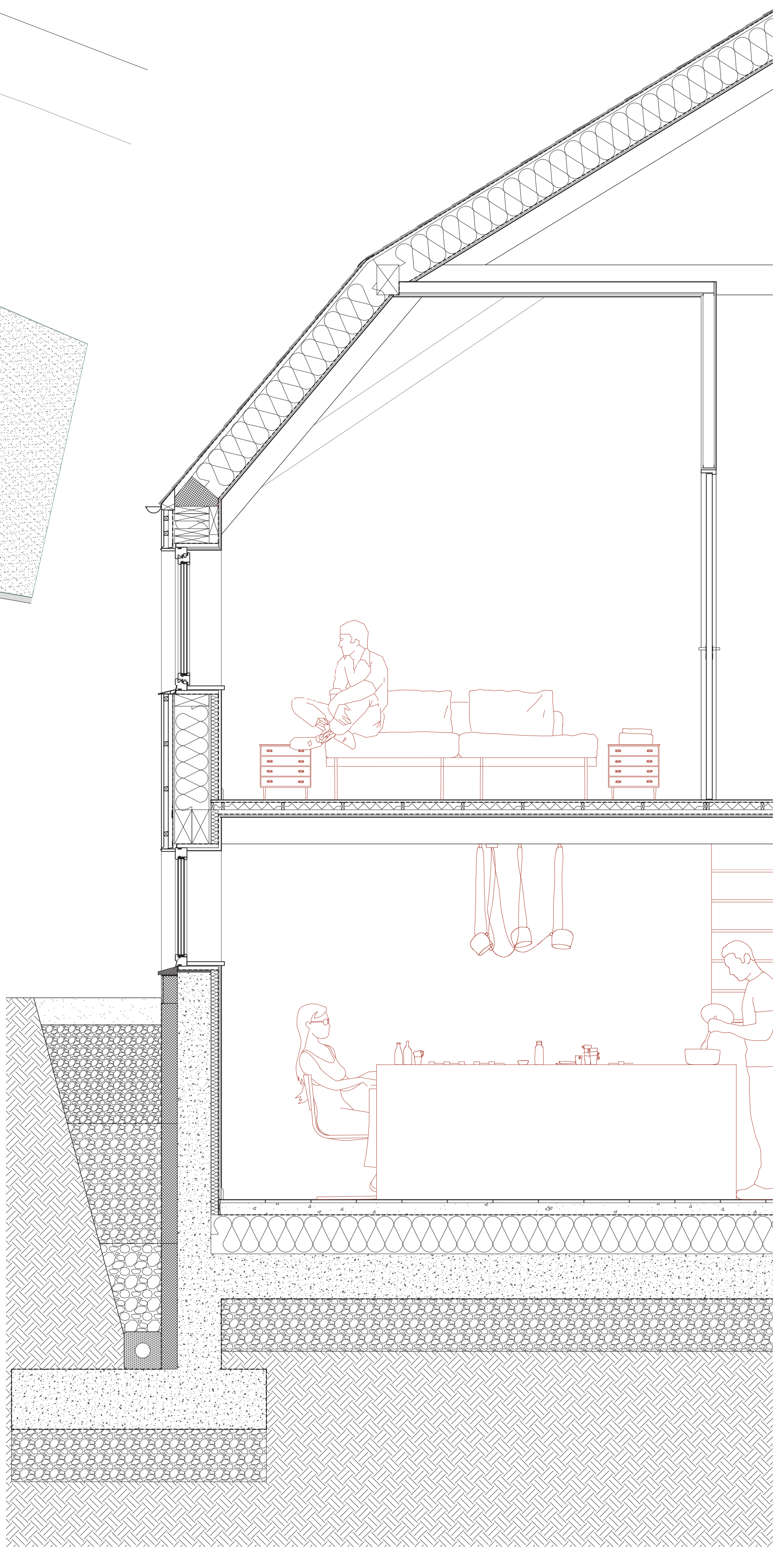
COUPE DÉTAIL - ÉCHELLE 1 : 20
