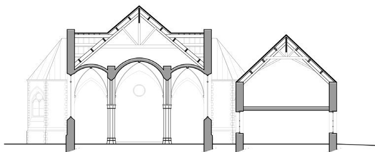
Coupe transversale
