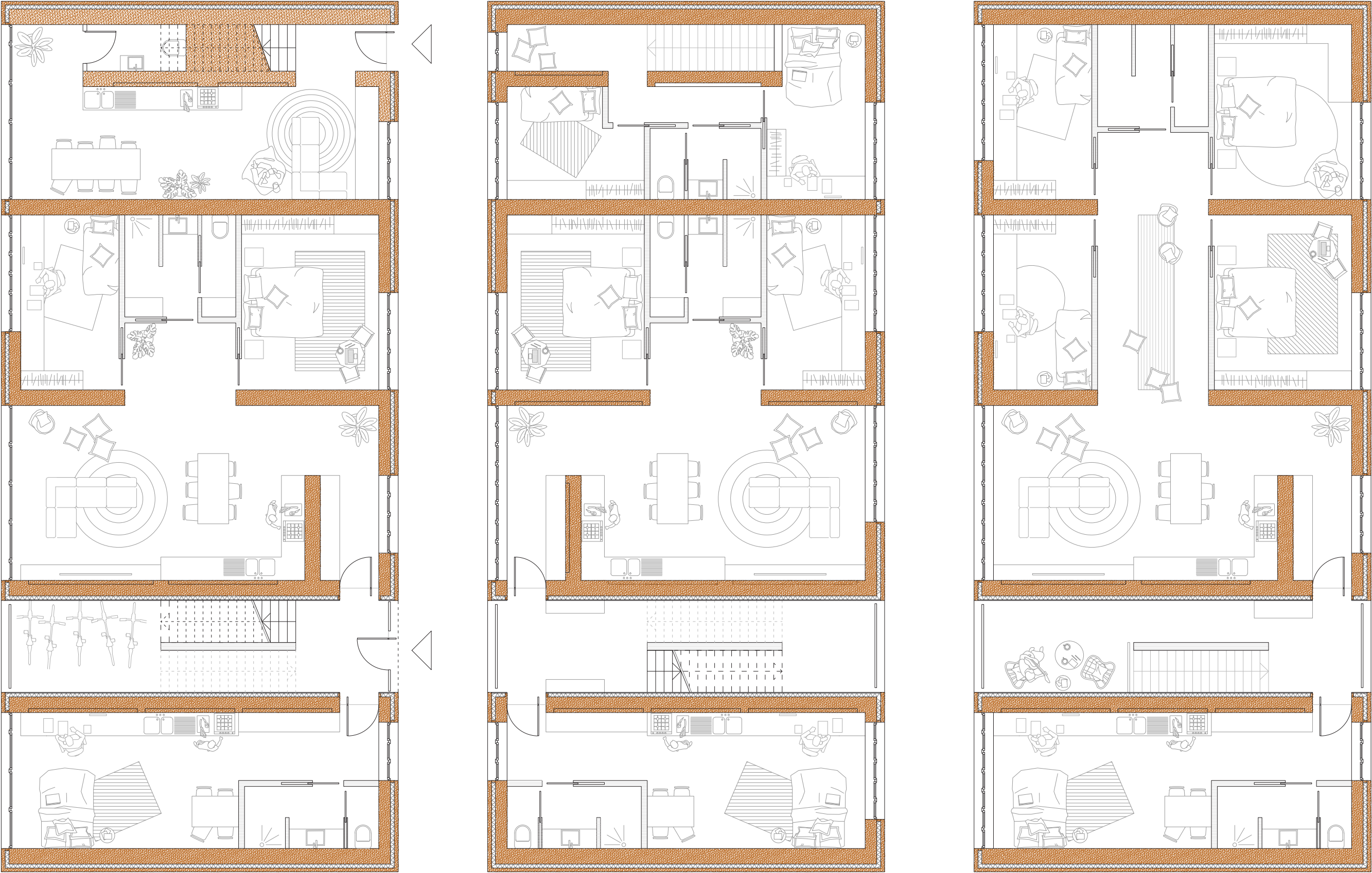
MODÈLE D'IMMEUBLE À APPARTEMENTS - PLAN
