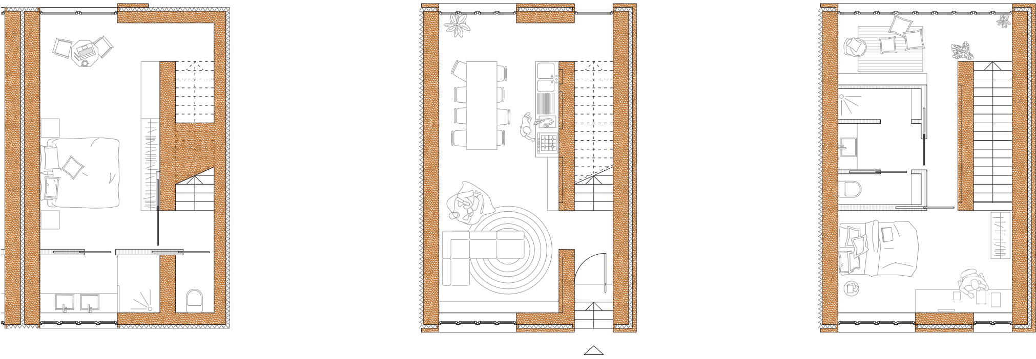
MODÈLE DE MAISON MITOYENNE - PLAN
