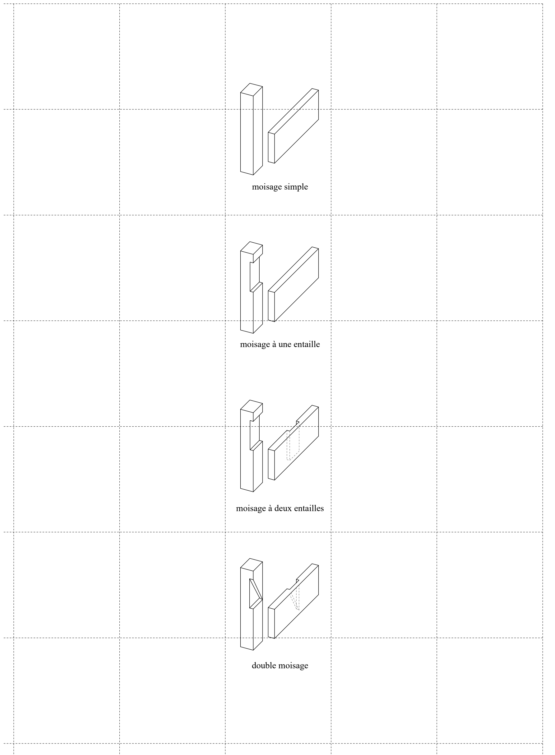
Assemblage des nœuds: moisage
