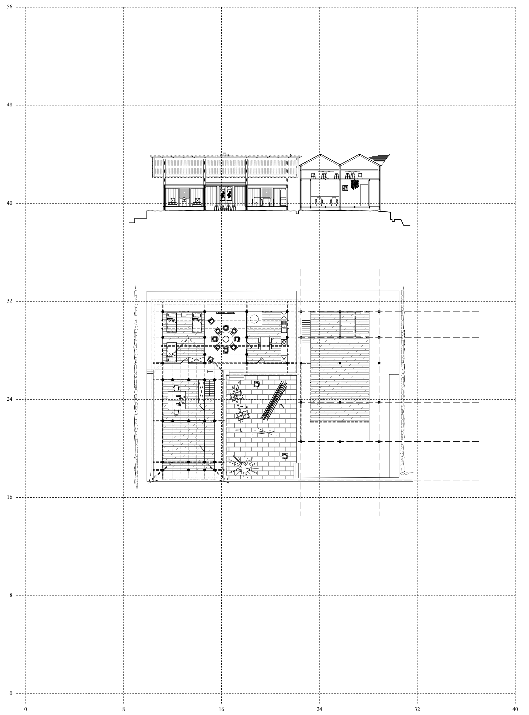
Plan et coupe d'implantation
