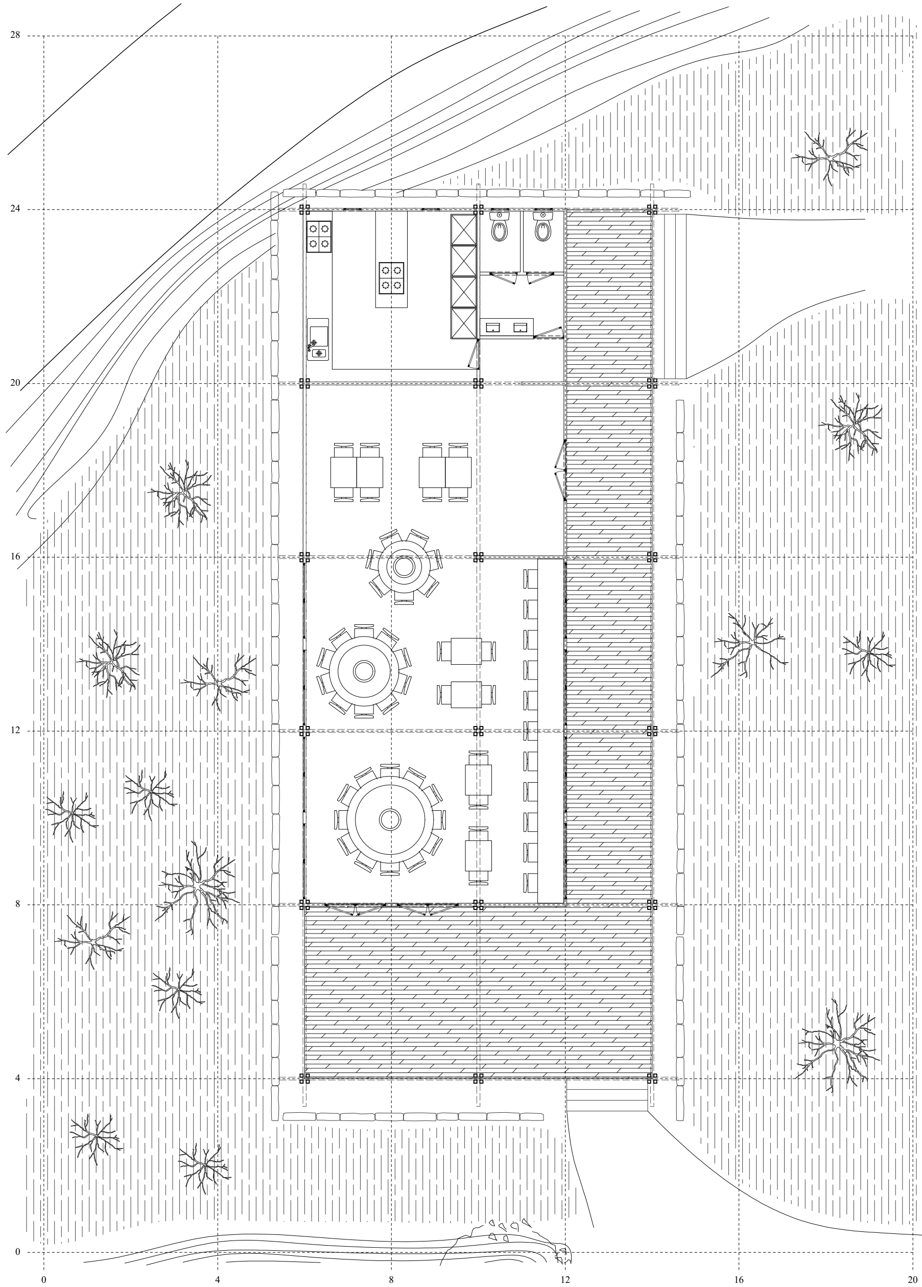
Plan détaillé
