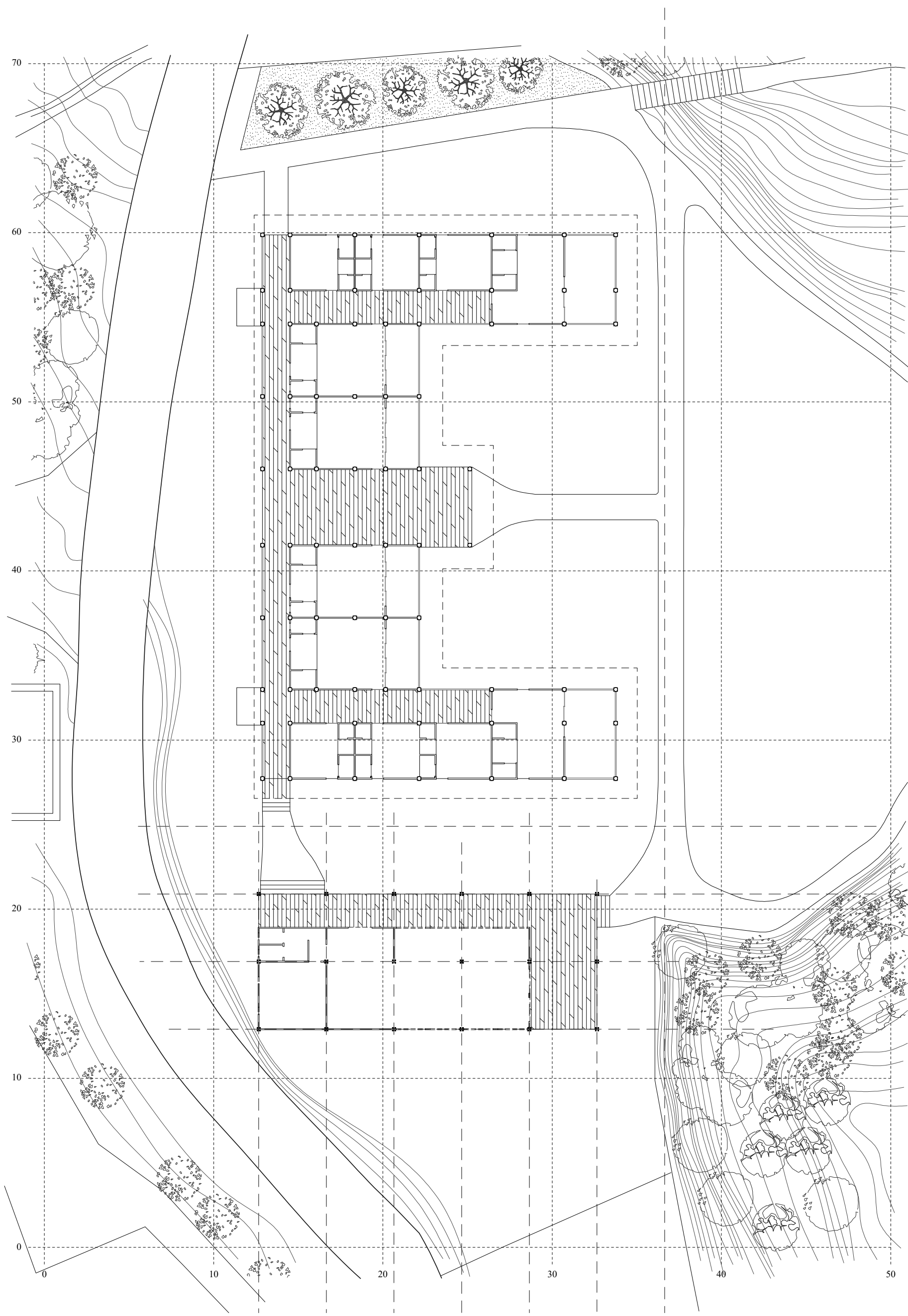
Plan d'implantation
