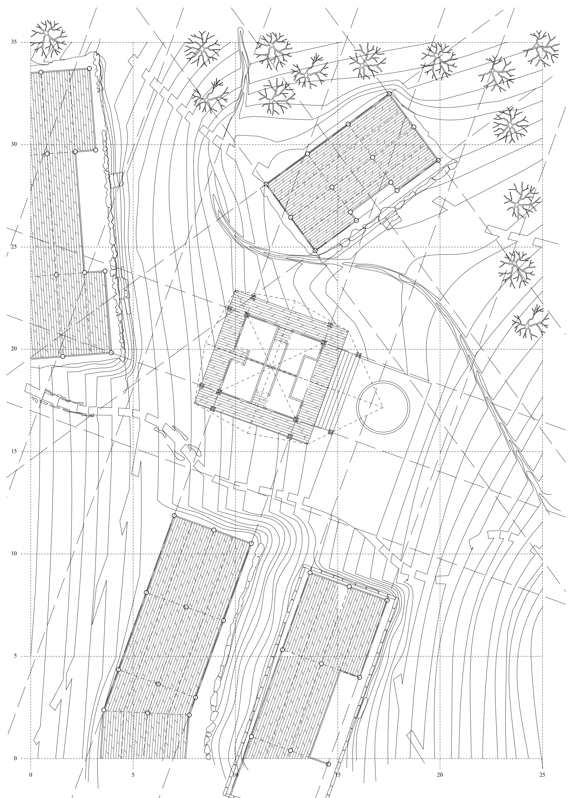
Plan d'implantation
