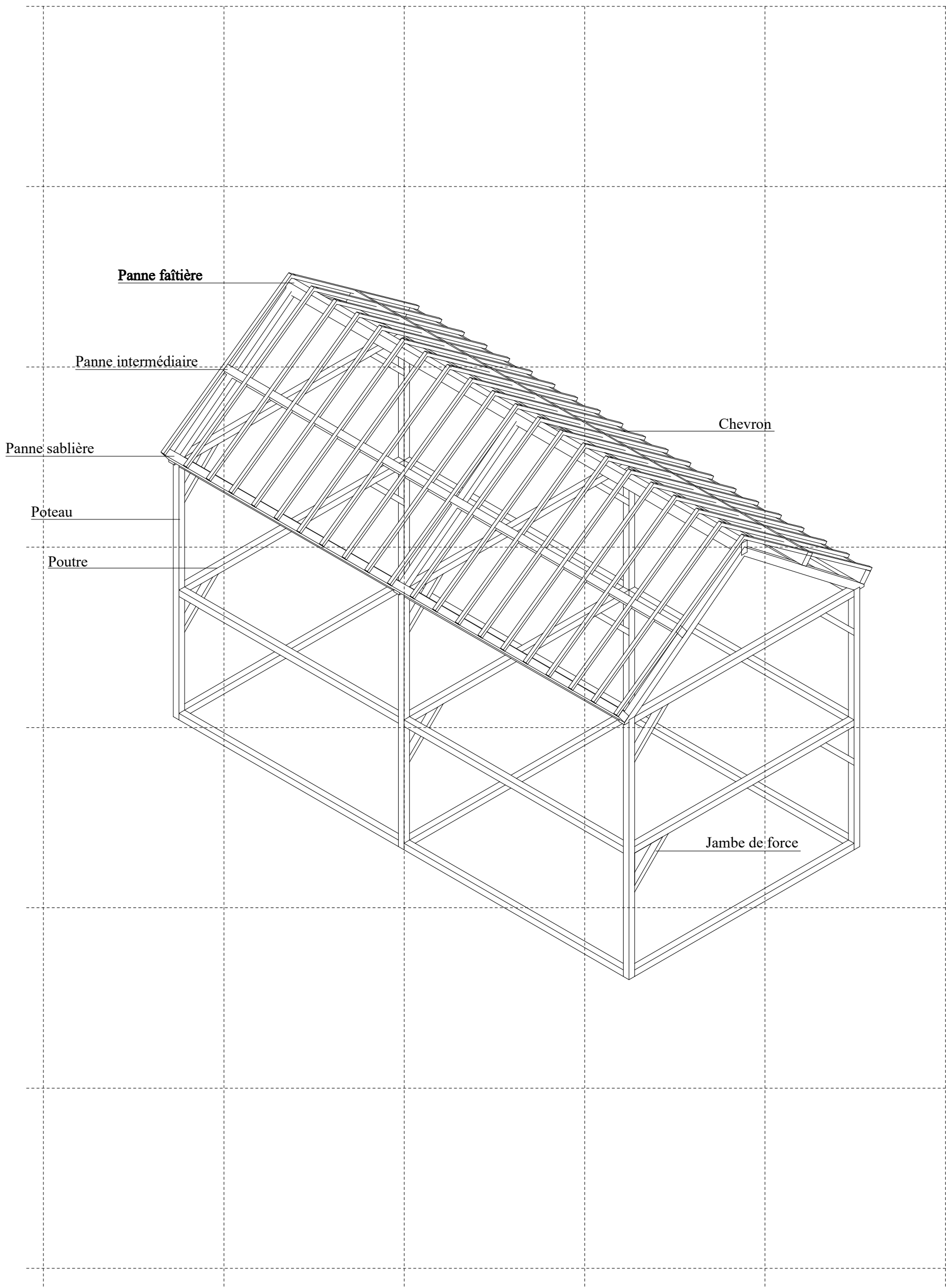
Système constructif: poteau-poutre
