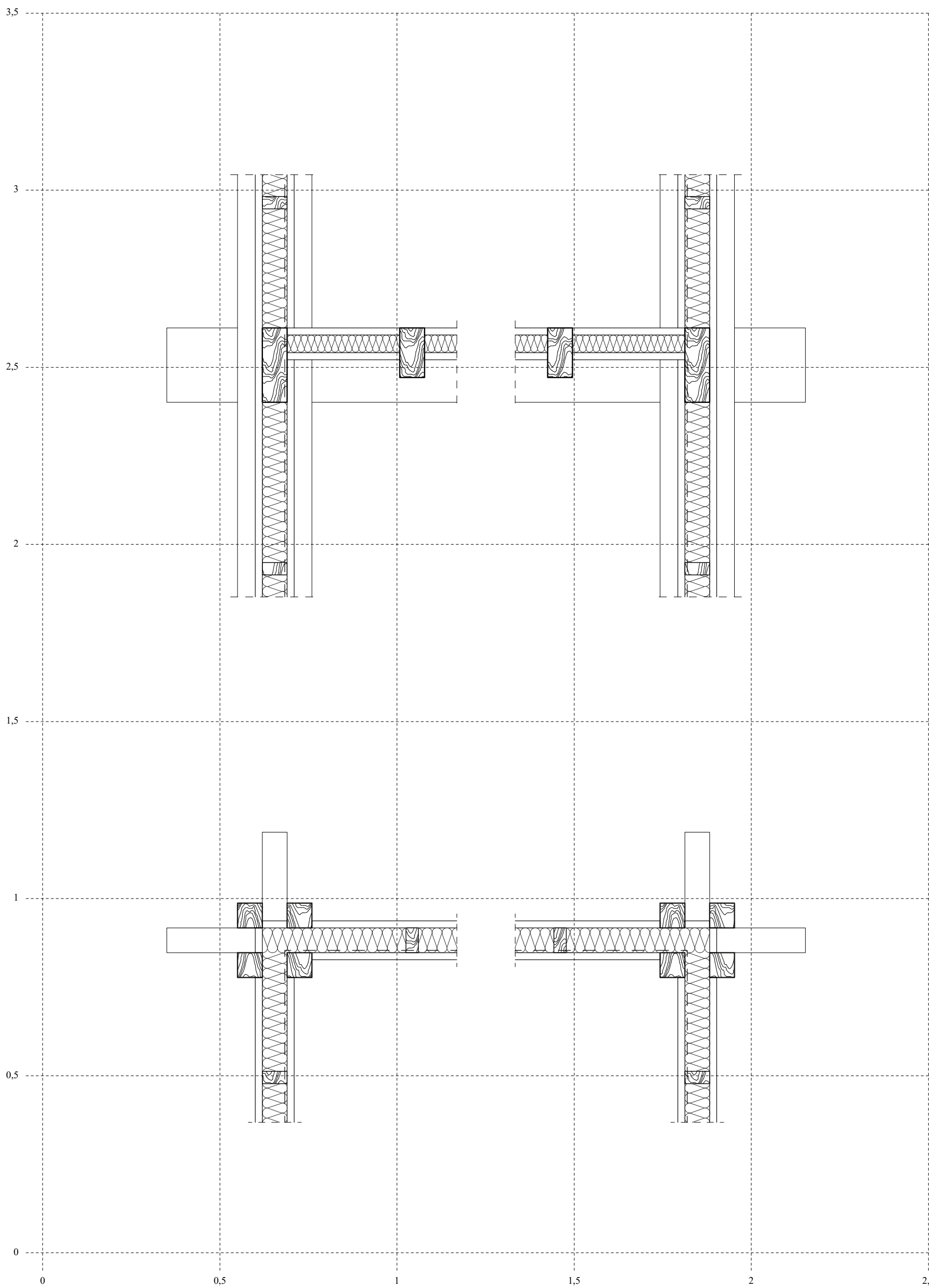
Détail technique
