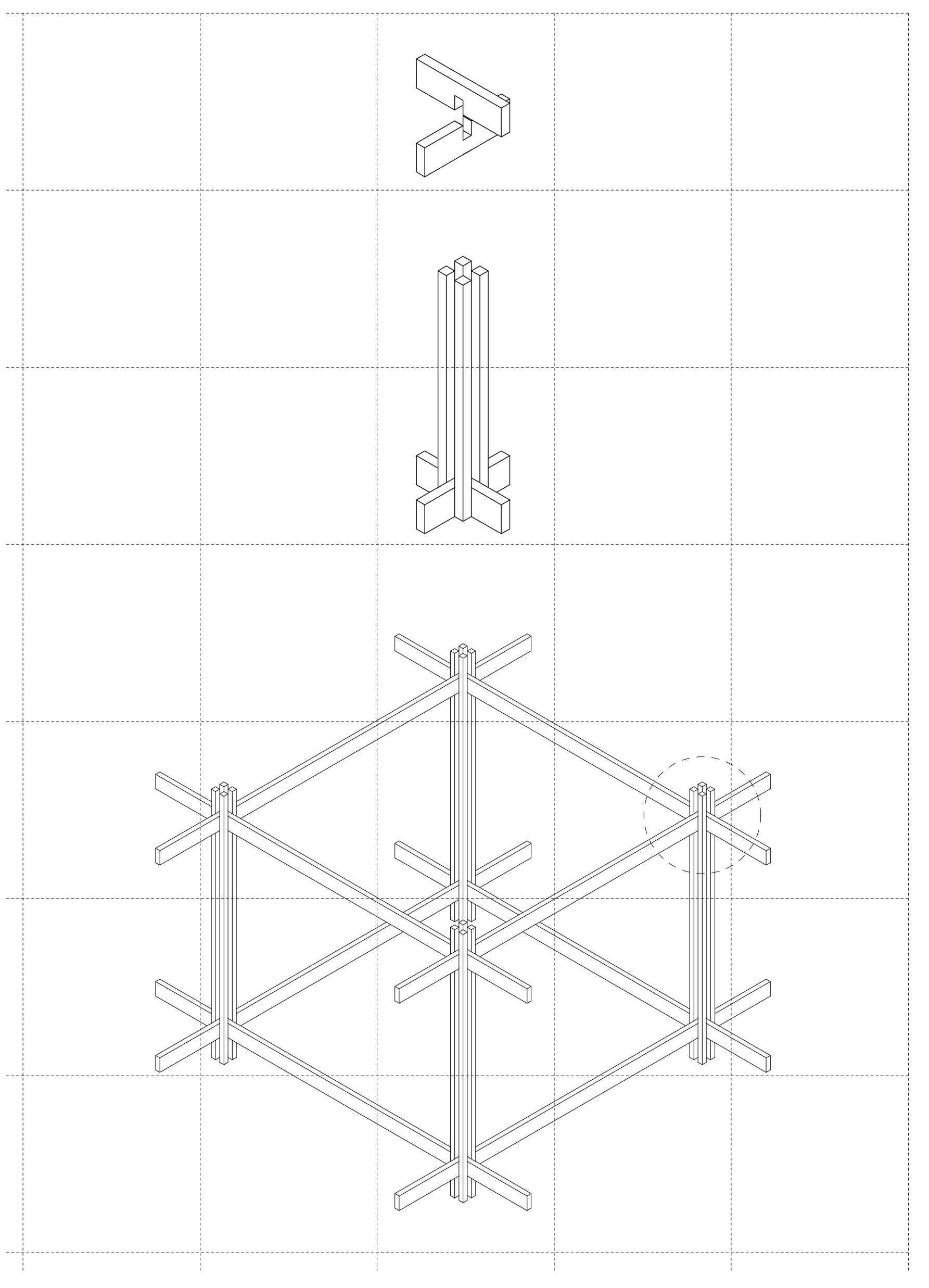
Axonométrie d'assemblage
