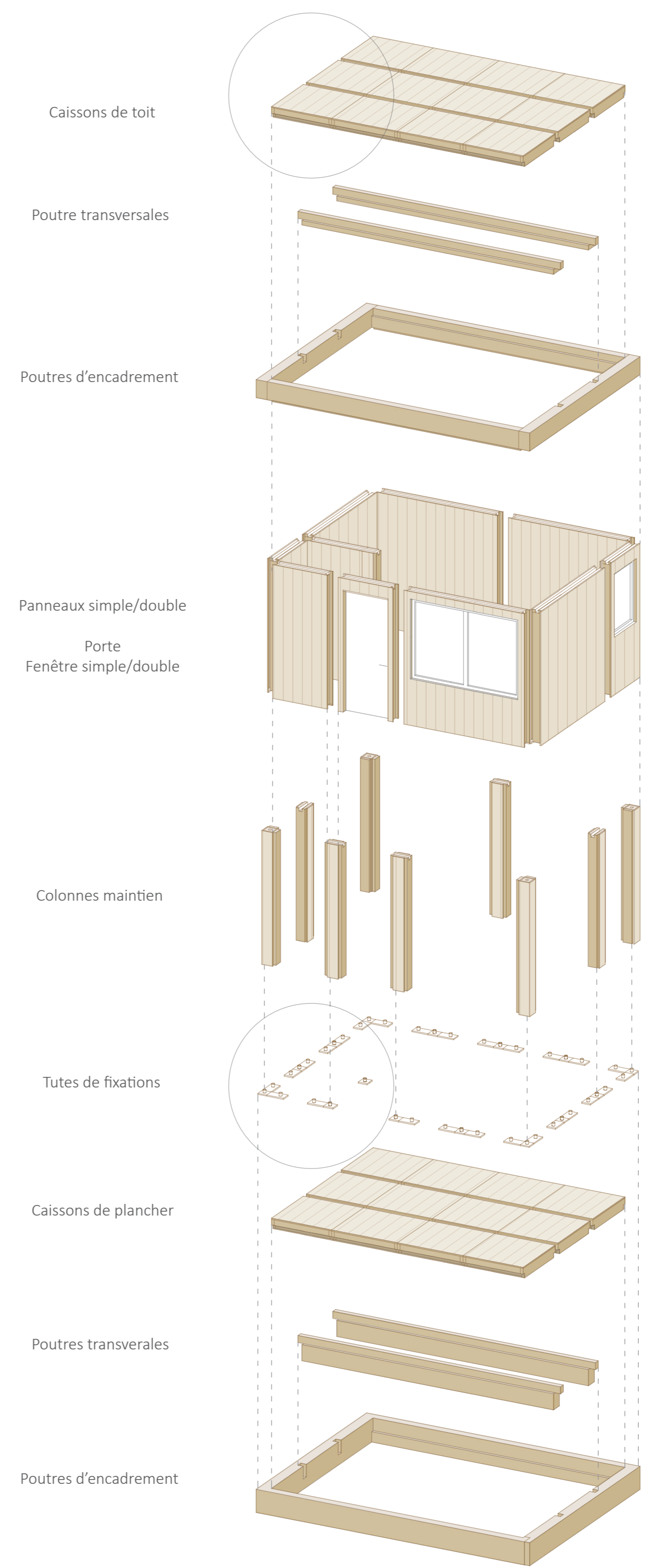
Assemblage complet d'un module
