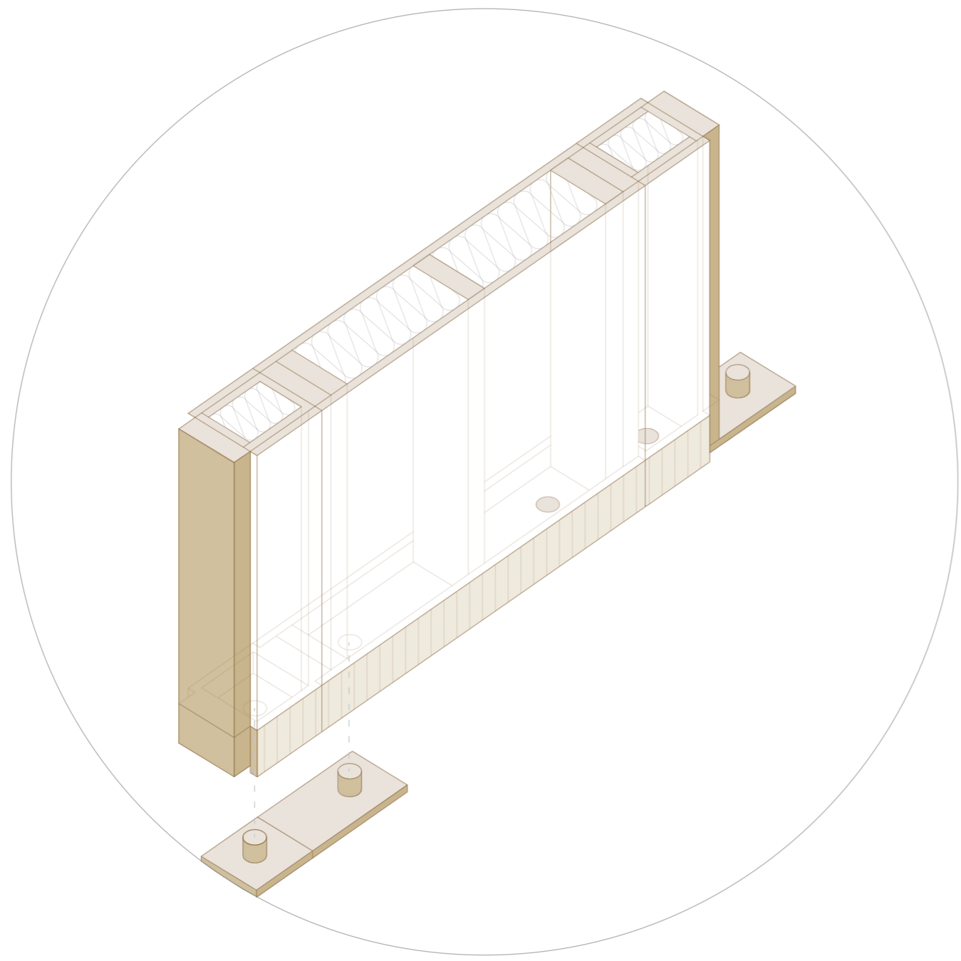
Détail assemblage panneaux
