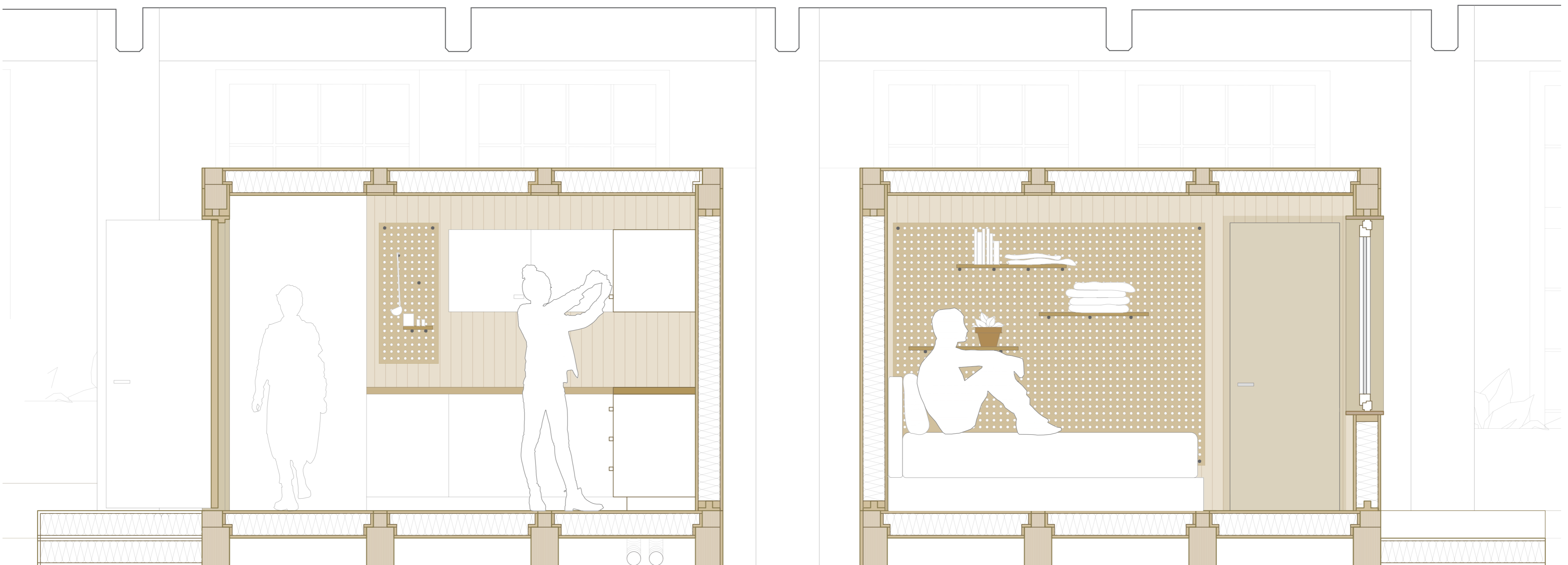
Coupe détail 1:20
