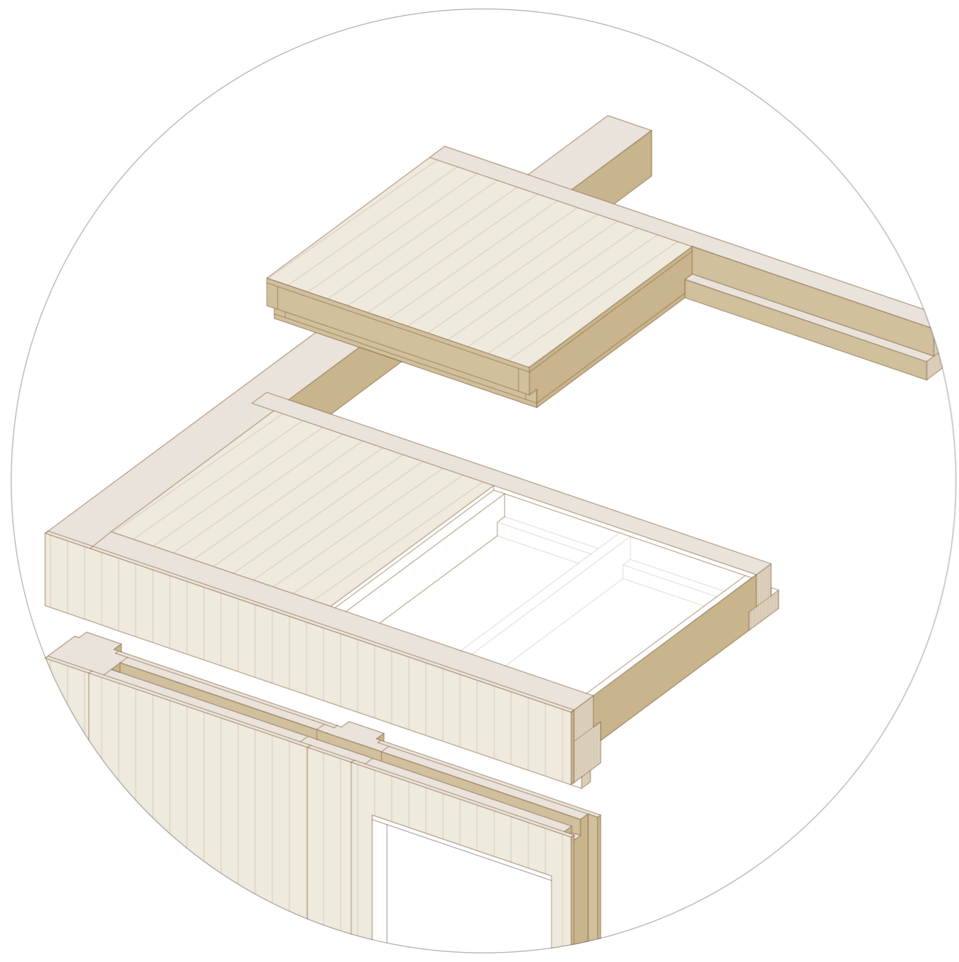
Détail assemblage toit
