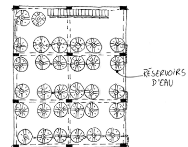
PLAN ÉTAGE +1
